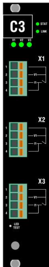
Рисунок 39 – Сторона подключения внешних цепей модуля C3.4
