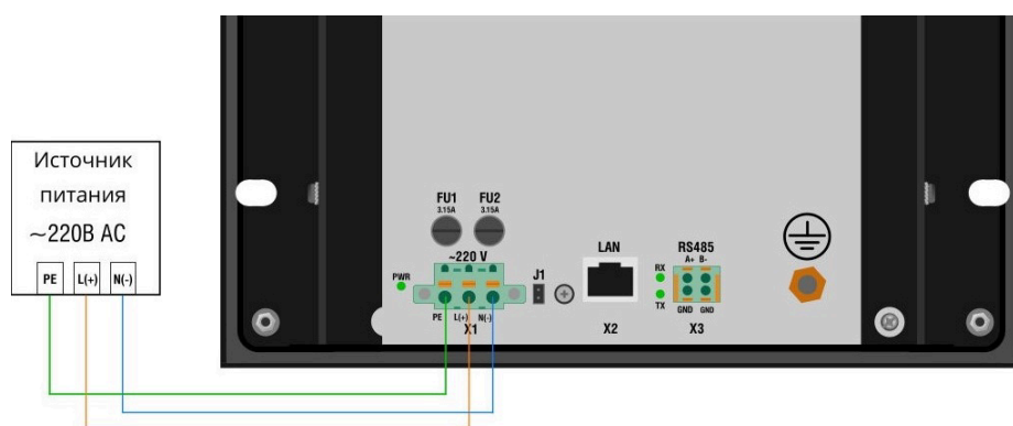
Рисунок 82 – Подключение выносного ИЧМ к сети постоянного или переменного тока 220 В
