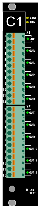
Рисунок 37 – Сторона подключения внешних цепей модуля C1.4
