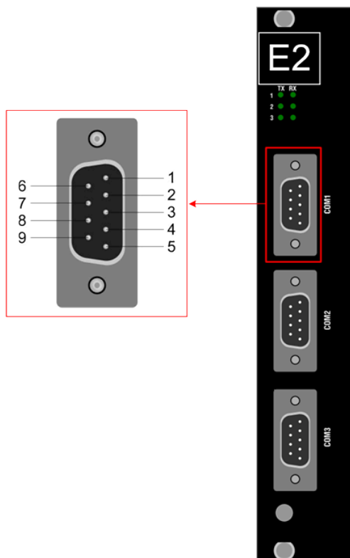
Рисунок 54 – Сторона подключения внешних цепей модуля E2.4
