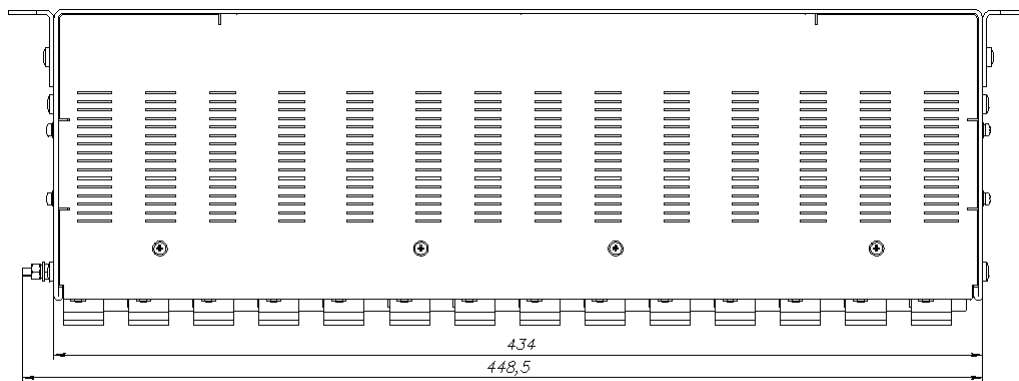
Рисунок Е.17 – Установочные размеры ARIS-2314, мм (вид сверху)
