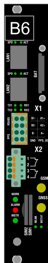
Рисунок 13 – Сторона подключения внешних цепей модуля В6.4
