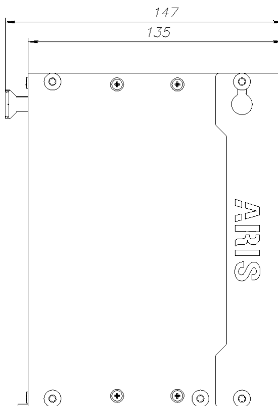
Рисунок Е.15 – Общий вид ARIS-2314
