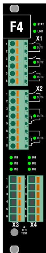
Рисунок 34 – Сторона подключения внешних цепей модуля F4.4
