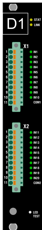
Рисунок 21 – Сторона подключения внешних цепей модуля D1.4
