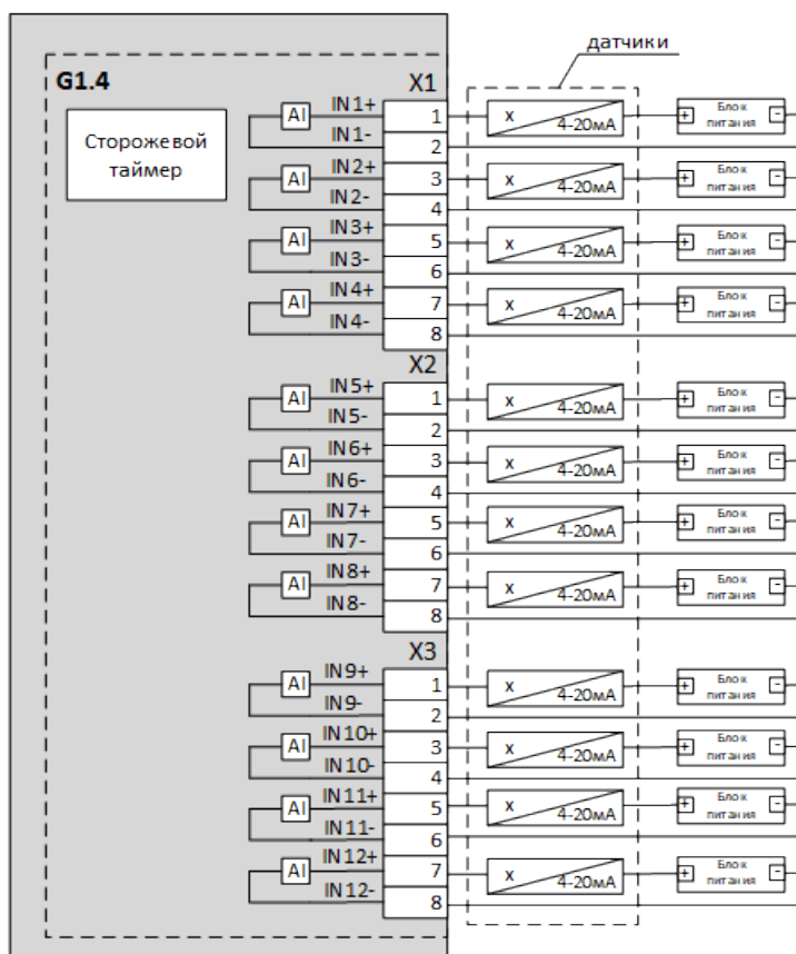
Рисунок 50 – Схема подключения внешних устройств к модулю G1.4
