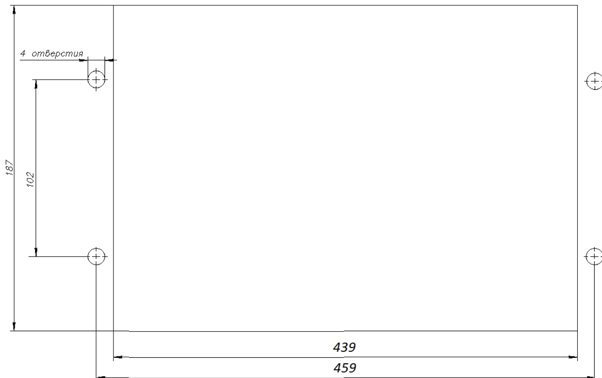
Рисунок Е.20 – Установочные размеры ARIS-2314 со встроенным ИЧМ, мм
