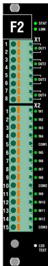
Рисунок 29 – Сторона подключения внешних цепей модуля F2.4
