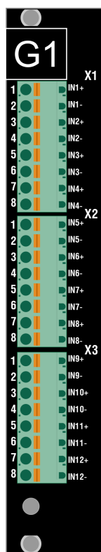
Рисунок 49 – Сторона подключения внешних цепей модуля G1.4
