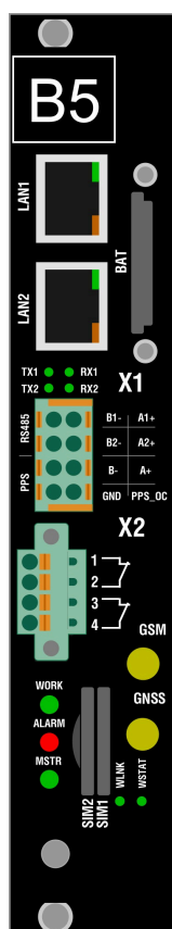
Рисунок 12 – Сторона подключения внешних цепей модуля В5.4
