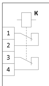
Рисунок 19 – Схема подключения реле LIVE контроля работоспособности устройства
