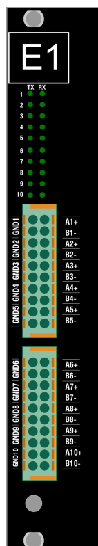
Рисунок 51 – Сторона подключения внешних цепей модуля E1.4
