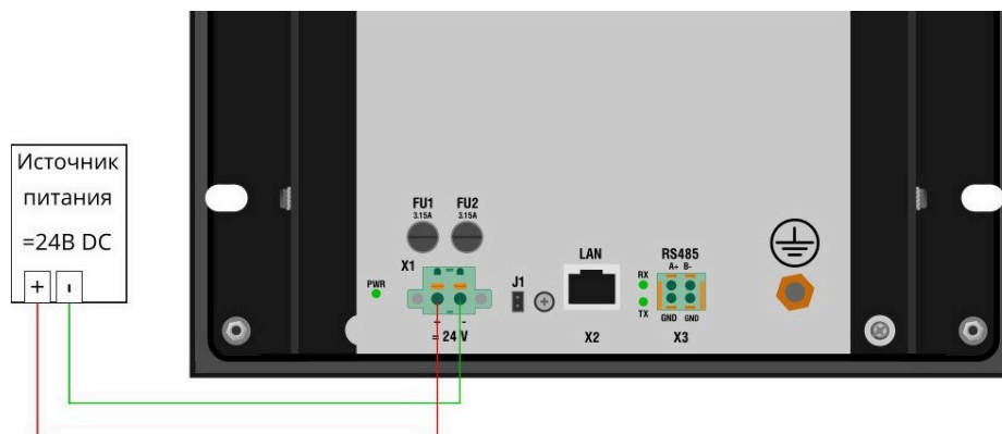
Рисунок 81 – Подключение выносного ИЧМ к сети постоянного тока 24 В
