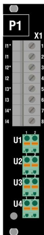
Рисунок 61 – Внешний вид стороны подключения внешних цепей модуля Р1.4 (Р2.4, Р3.4, Р4.4)
