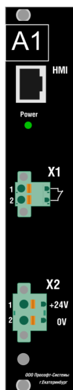
Рисунок 2 – Сторона подключения внешних цепей модуля А1.4
