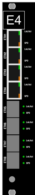
Рисунок 59 – Сторона подключения внешних цепей модуля E4.4
