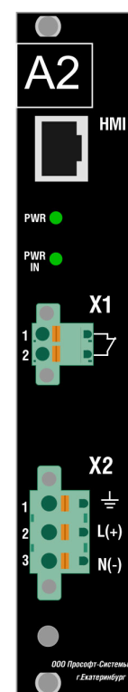
Рисунок 3 – Сторона подключения внешних цепей модуля А2.4
