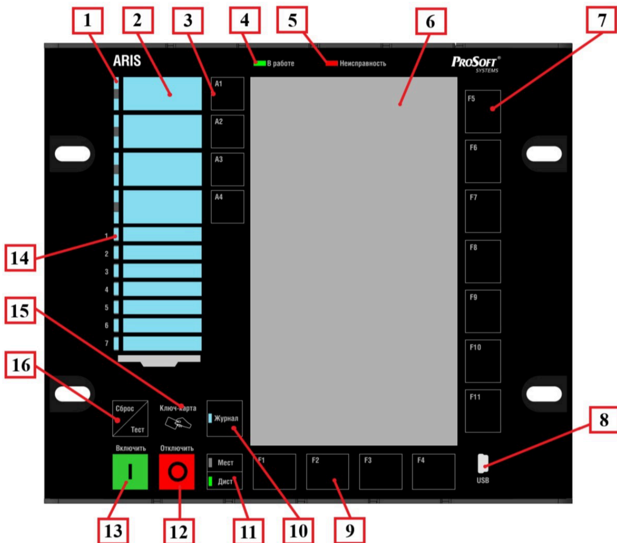
Рисунок 83 – Элементы лицевой панели модуля ИЧМ
