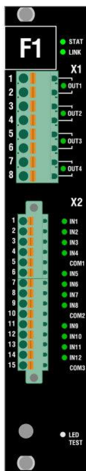
Рисунок 27 – Сторона подключения внешних цепей модуля F1.4
