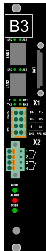
Рисунок 11 – Сторона подключения внешних цепей модуля В3.4
