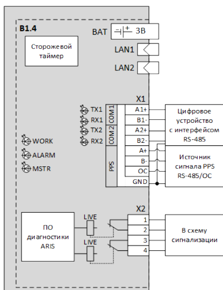
Рисунок 14 – Схема подключения модуля В1.4 Рисунок 15 – Схема подключения модуля В3.4
