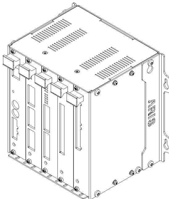
Рисунок Е.1 – Общий вид ARIS-2305
