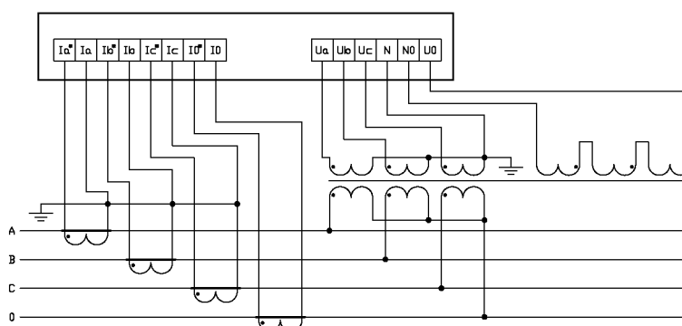
Рисунок И.5 – Схема подключения модулей М4.4 к четырехпроводной сети 4ТТ и 3 ТН 0 , заземленная нейтраль и обмотка 3U 0
