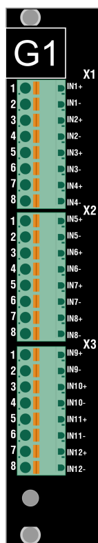
Рисунок 49 – Сторона подключения внешних цепей модуля G1.4
