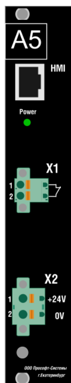
Рисунок 6 – Сторона подключения внешних цепей модуля A5.4
