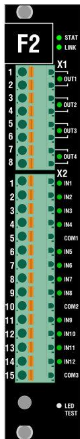
Рисунок 29 – Сторона подключения внешних цепей модуля F2.4
