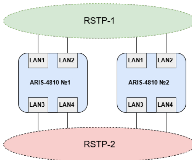
Рисунок 242 – Схема поддержки нескольких экземпляров RSTP одним ARIS-4810
