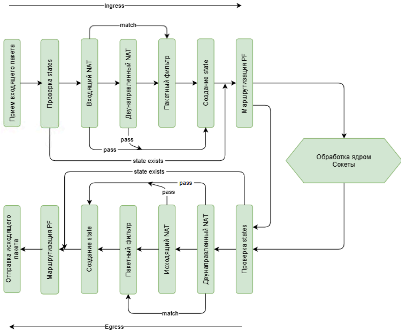
Рисунок 264 – Блок-схема конвейера обработки ip-пакетов
