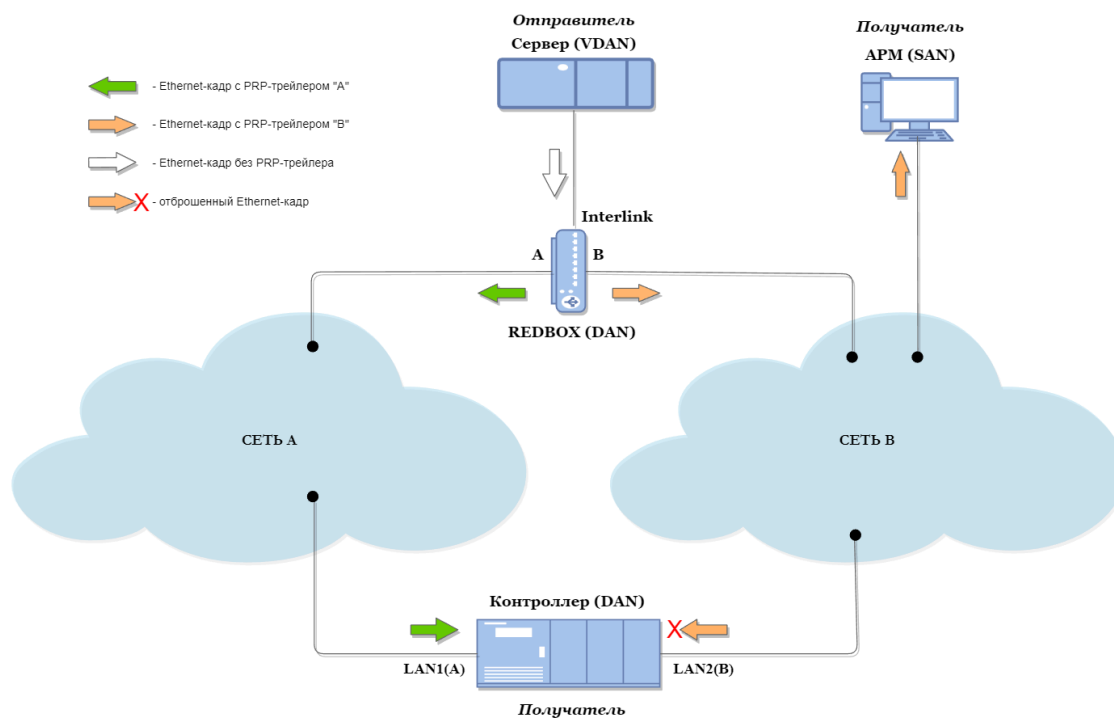
Рисунок 231 – Представление алгоритма работы в режиме резервирования «PRP»
