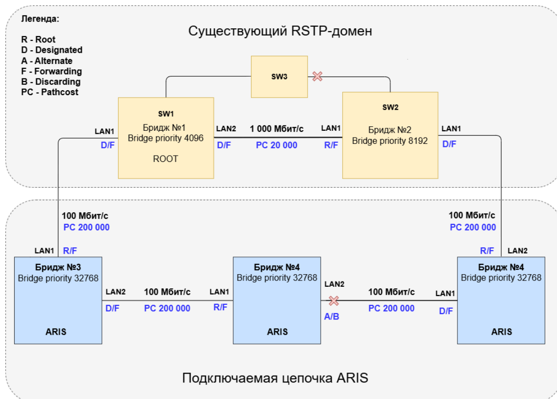
Рисунок 241 – Схема подключения цепочки из ARIS
