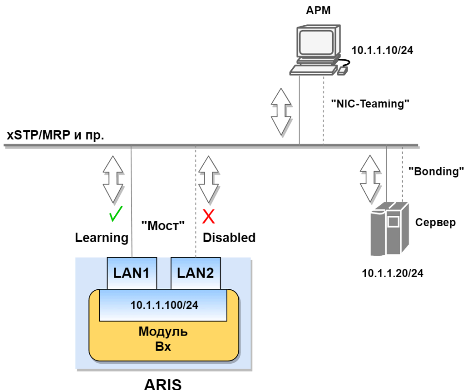
Рисунок 233 – Представление алгоритма работы в режиме «Горячий резерв»
