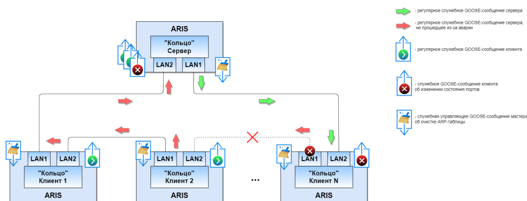
Рисунок 234 – Представление алгоритма работы в режиме «Кольцо»
