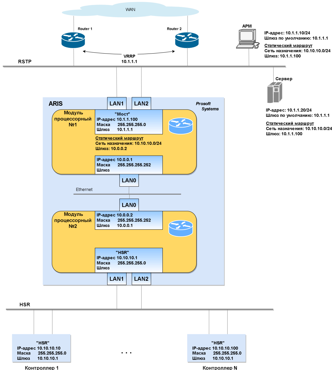
Рисунок 246 – Пример использования второго процессорного модуля в качестве шлюза
