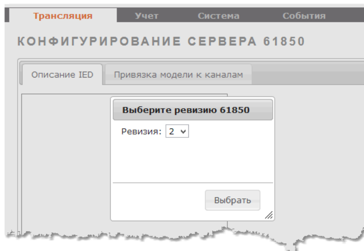
Рисунок 67 – Запрос на выбор ревизии сервера МЭК 61850-8-1
