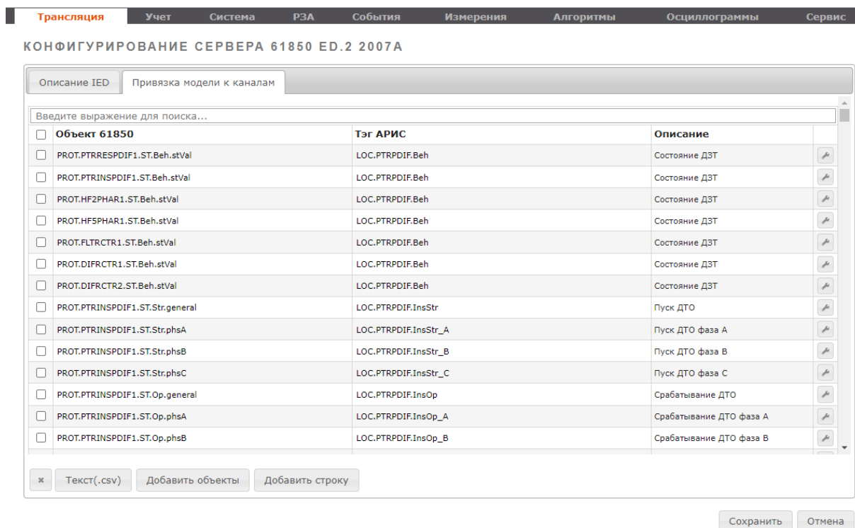
Рисунок 80 – Вкладка для редактирования привязки текущей модели IED к каналам сервера МЭК 61850–8–1
