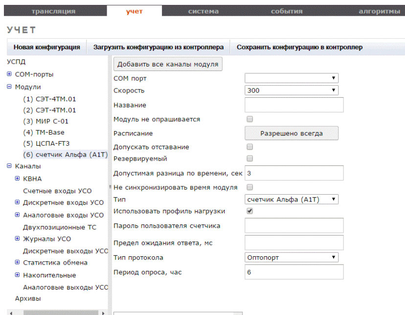
Рисунок 208 – Редактирование параметров модуля УСД
