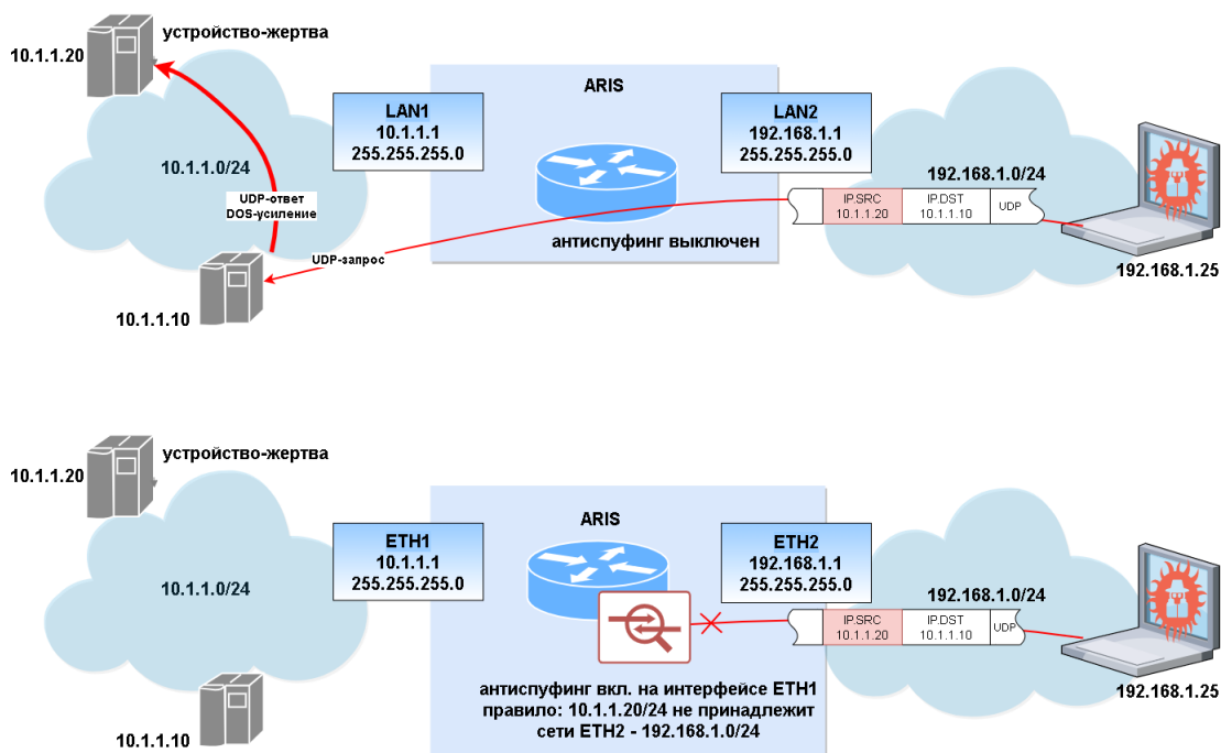
Рисунок 266 – Поясняющие схемы для правила 1
