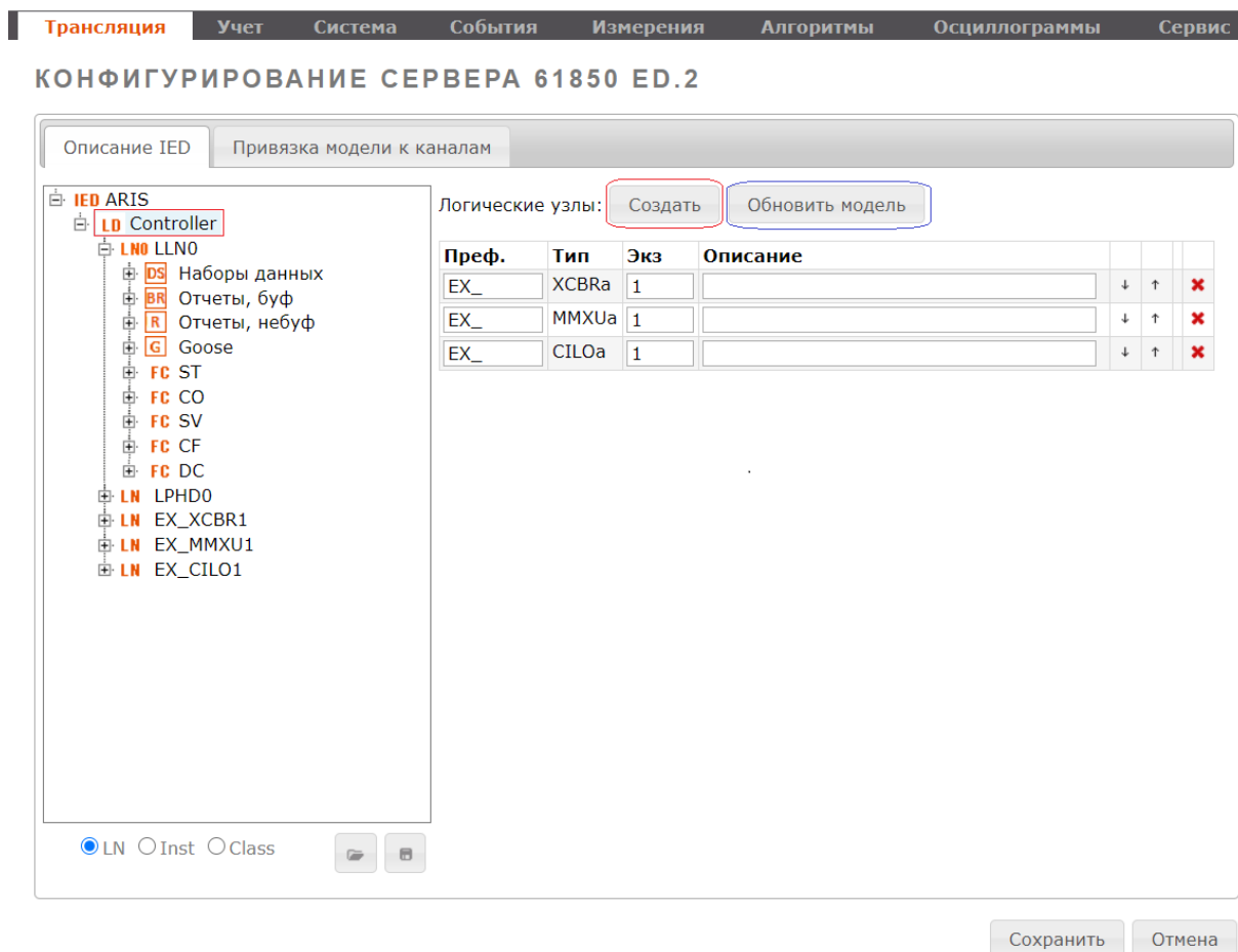
Рисунок 69 – Узел «Controller» в структуре IED
