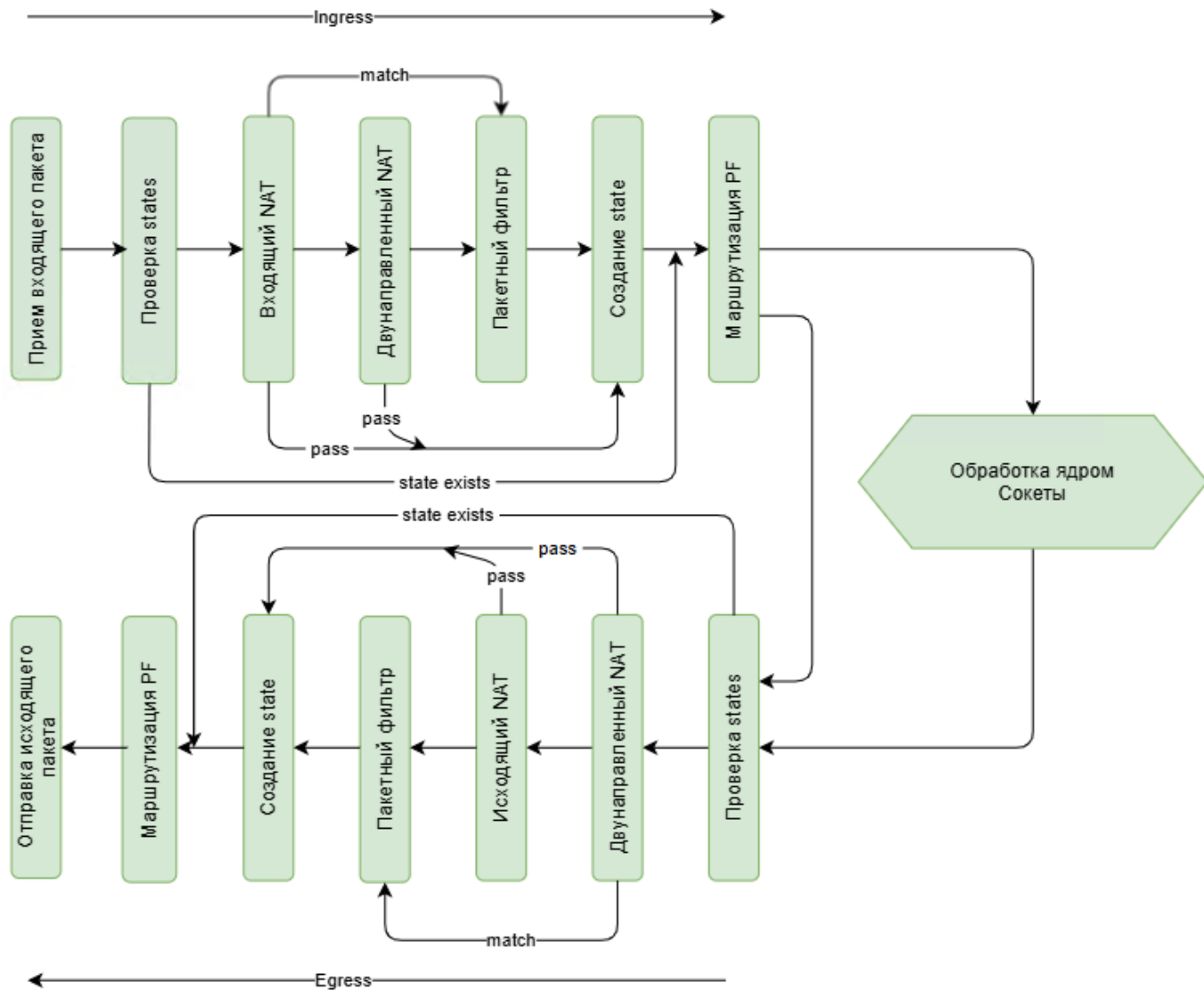
Рисунок 263 – Блок-схема конвейера обработки ip-пакетов
