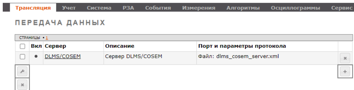
Рисунок 97 – Добавление сервера DLMS_COSEM
