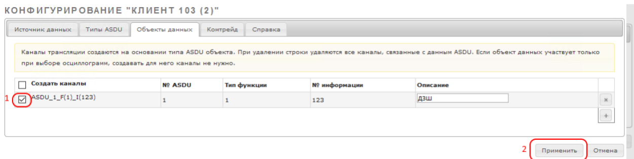
Рисунок 157 – Добавление клиента в трансляцию
