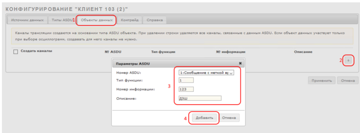
Рисунок 156 – Создание канала ТС
