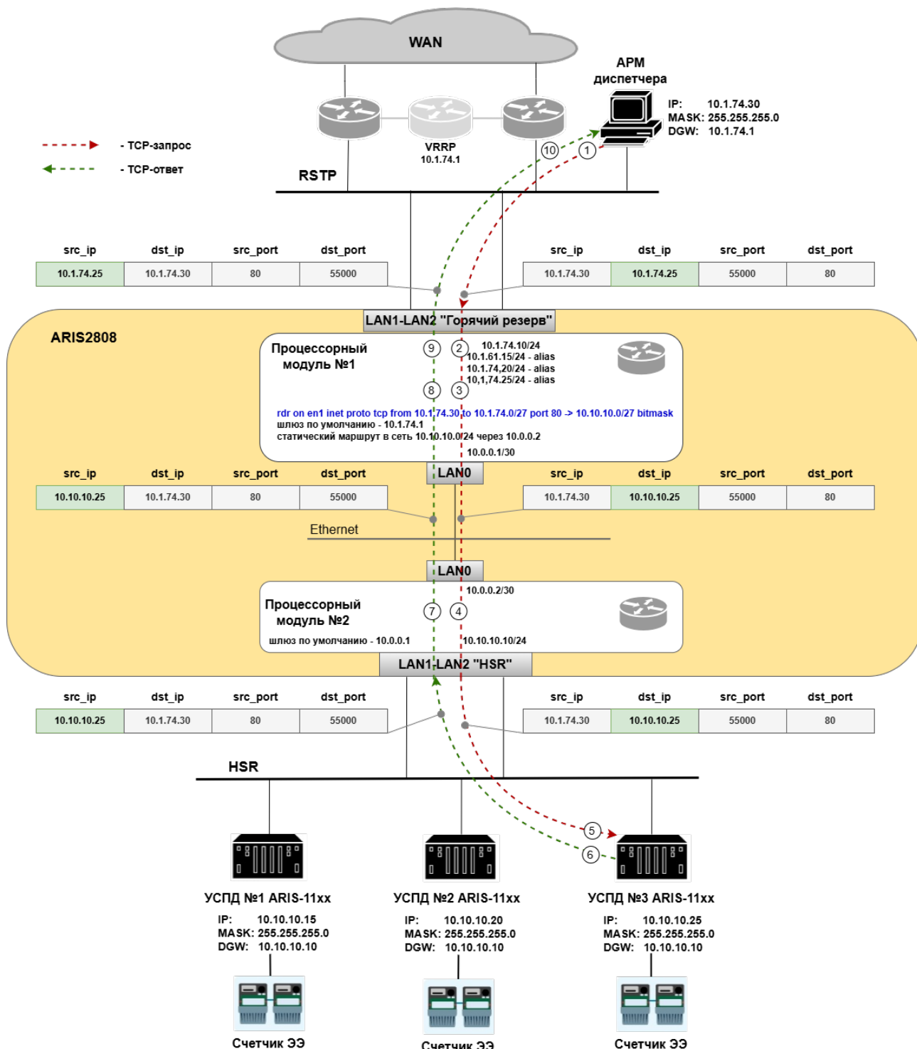
Рисунок 272 – Пример подключения АРМ диспетчера к УСПД со входящим NAT
