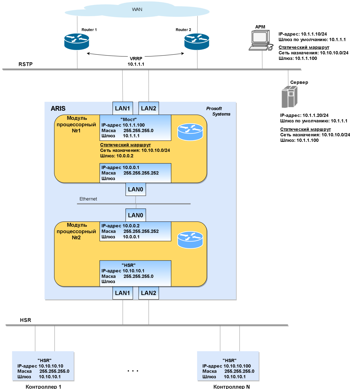
Рисунок 245 – Пример использования второго процессорного модуля в качестве шлюза
