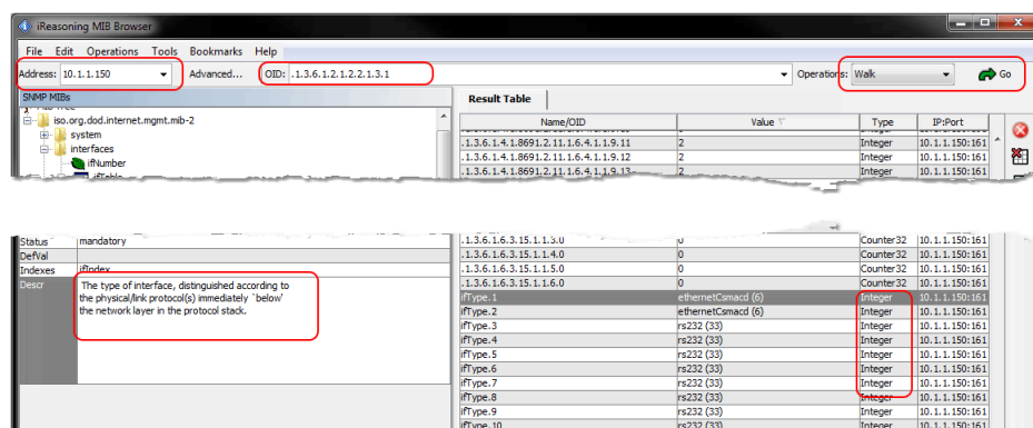
Рисунок 139 – Отображение OID с помощью утилиты «MIB Browser»
