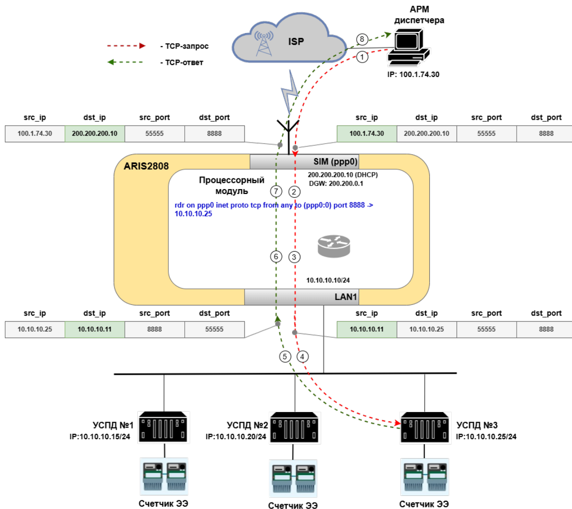
Рисунок 274 – Пример настройки входящего NAT для SIM-интерфейса
