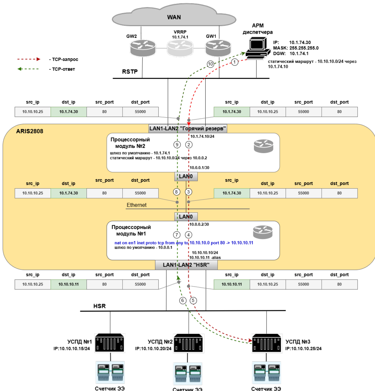
Рисунок 273 – Пример подключения АРМ диспетчера к УСПД с исходящим NAT
