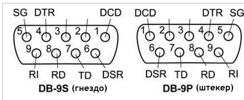
Рисунок 56 – Схема подключения RS-232 Sync
