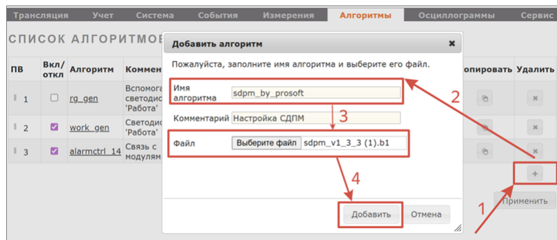
Рисунок 307 – Добавление алгоритма
