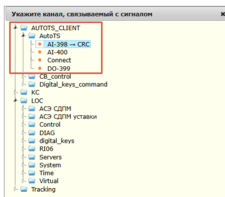
Рисунок 312 – Привязка канала
