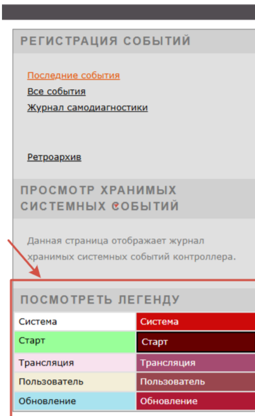
Рисунок 314 – Просмотр легенды
