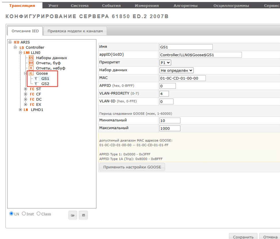
Рисунок 78 – Отображение «GOOSE-сообщения» в дереве IED
