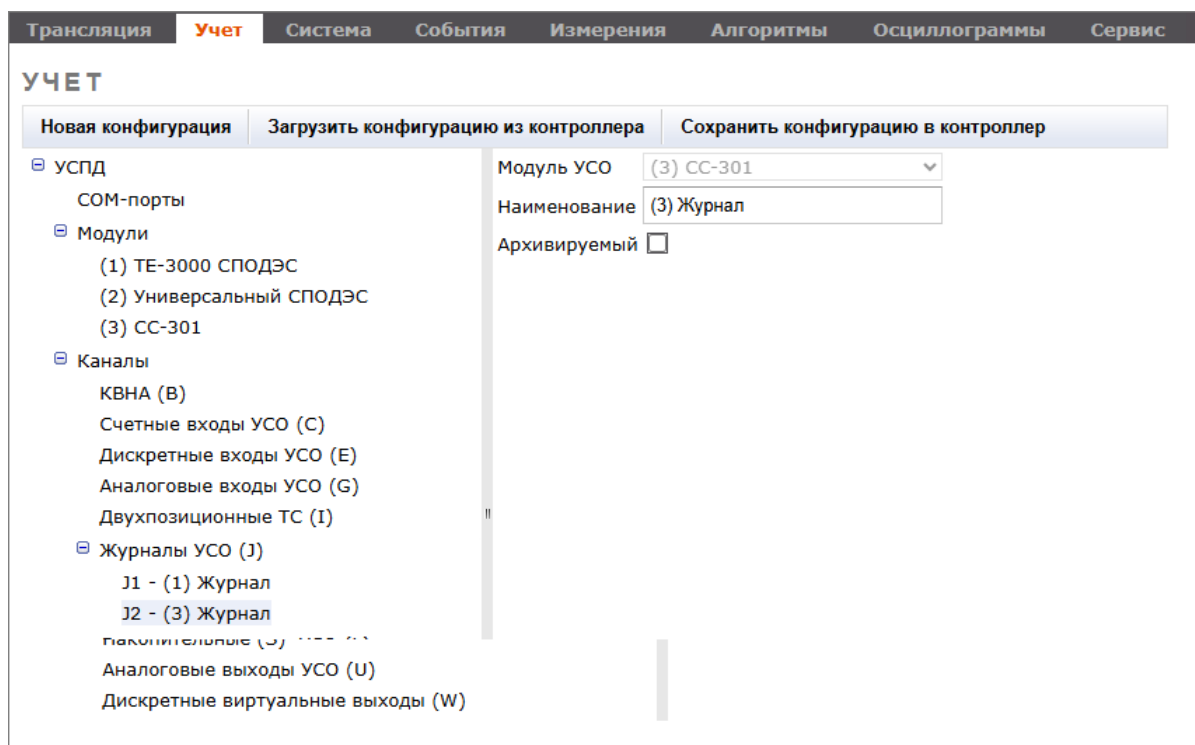
Рисунок 223 – Настройка журнального канала
