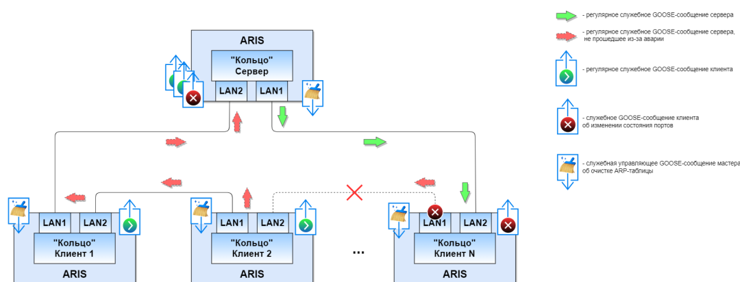
Рисунок 233 – Представление алгоритма работы в режиме «Кольцо»
