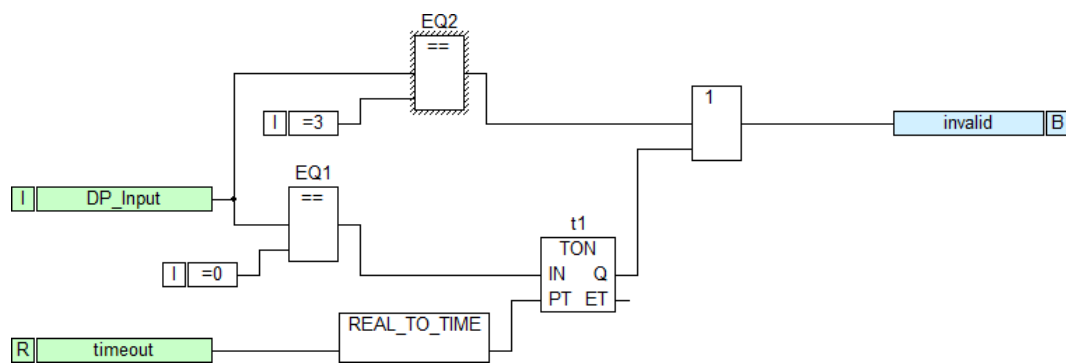
Рисунок 331 – Алгоритм контроля состояния КА
