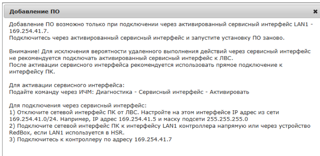
Рисунок 250 – Окно предупреждения активации сервисного интерфейса
