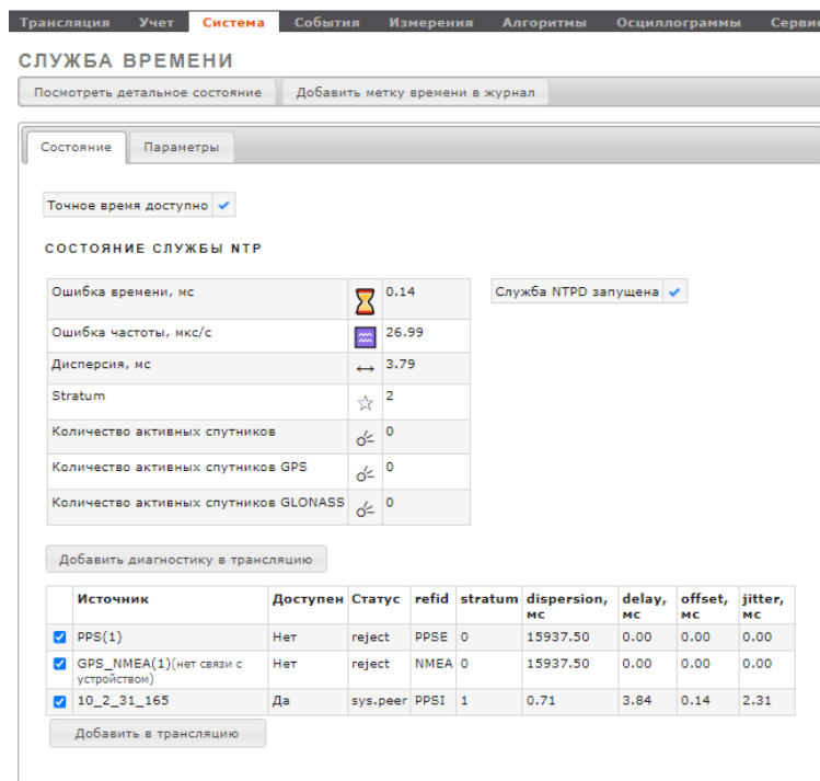
Рисунок 251 – Служба времени. Вкладка «Состояние»
