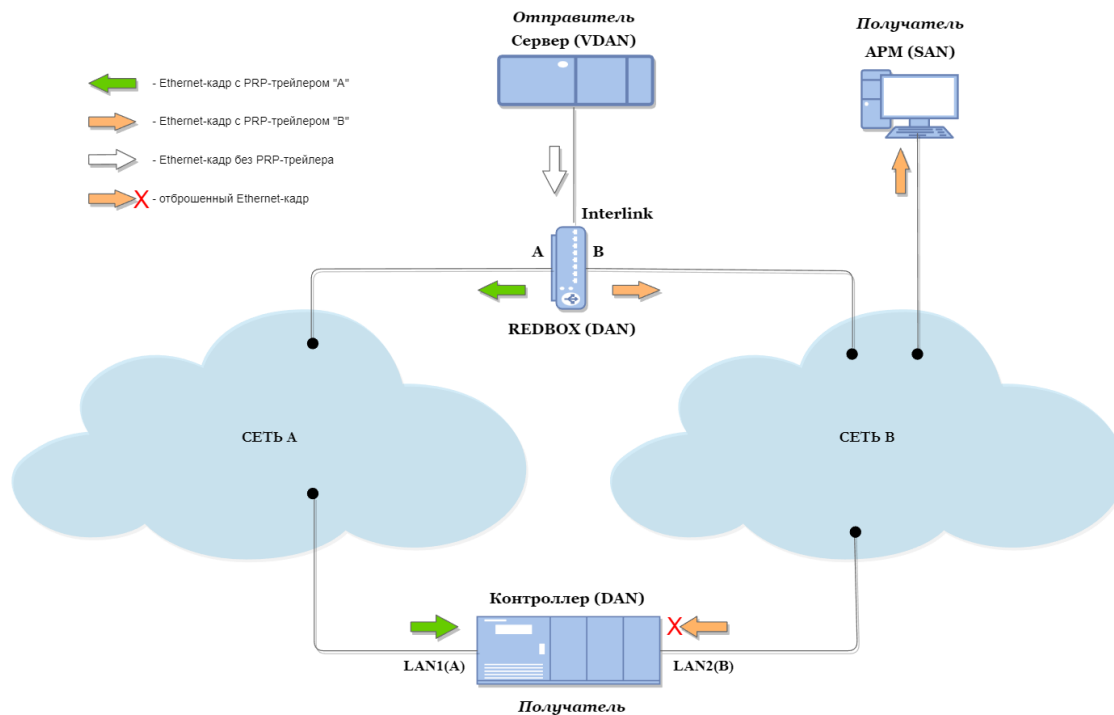
Рисунок 230 – Представление алгоритма работы в режиме резервирования «PRP»
