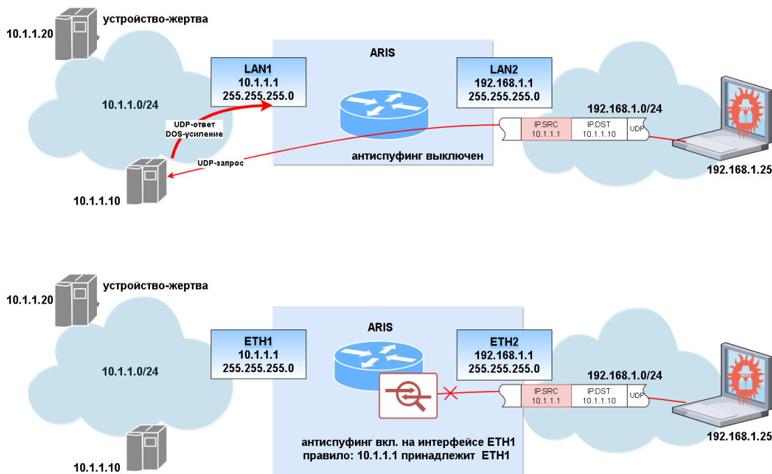
Рисунок 267 – Поясняющие схемы для правила 2
