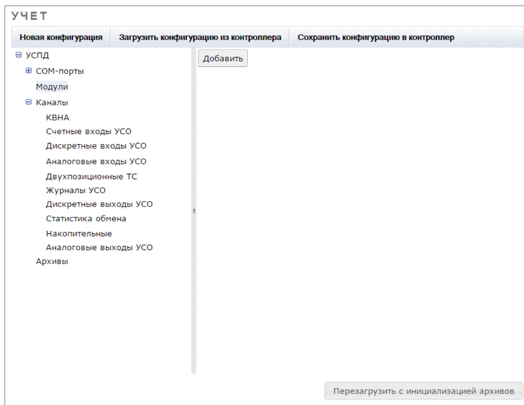
Рисунок 191 – Форма конфигурирования счетчиков
