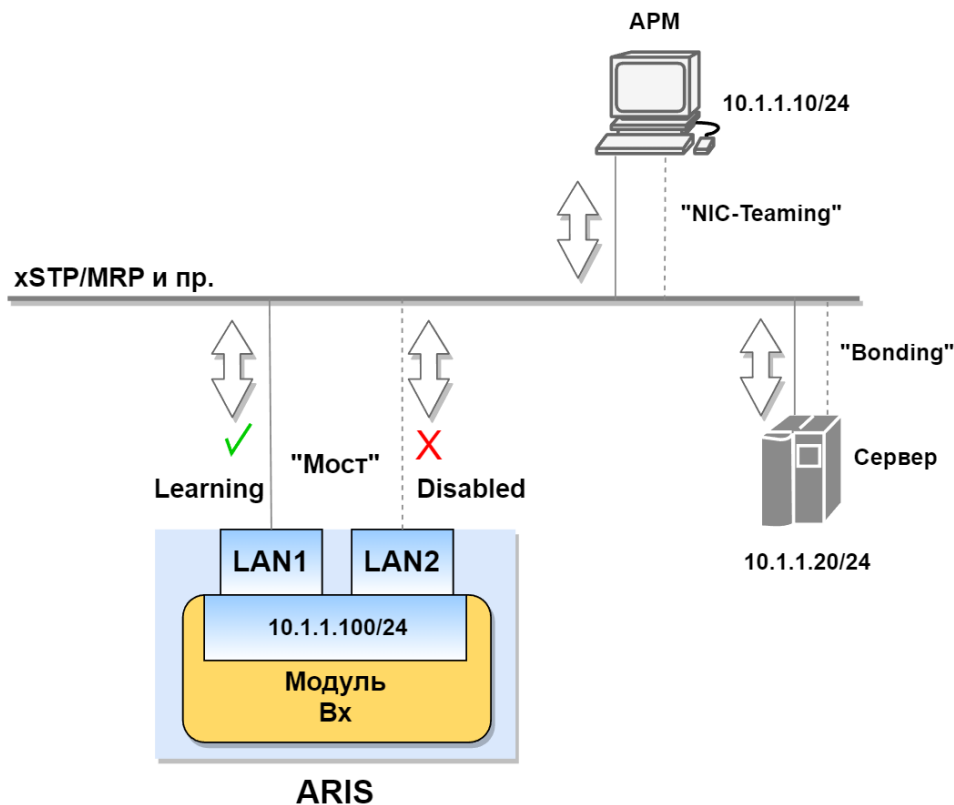
Рисунок 232 – Представление алгоритма работы в режиме «Горячий резерв»
