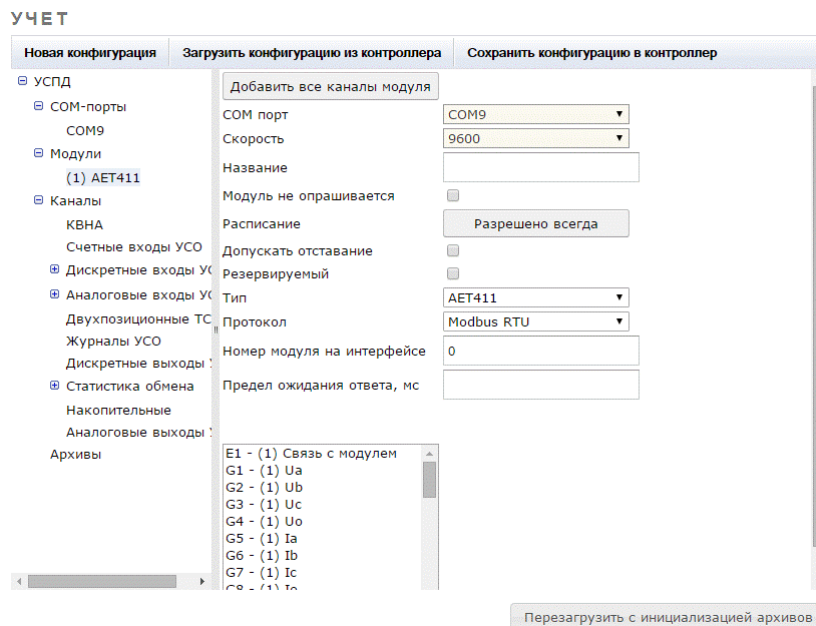
Рисунок 205 – Форма конфигурирования модулей УСО
