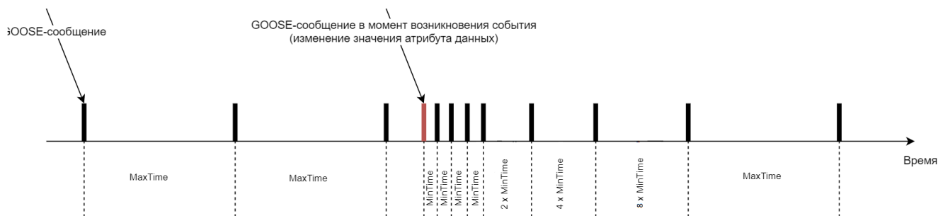
Рисунок 75 – Диаграмма публикации GOOSE-сообщения
