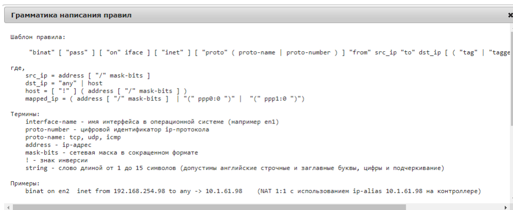
Рисунок 271 – Грамматика написания правил
