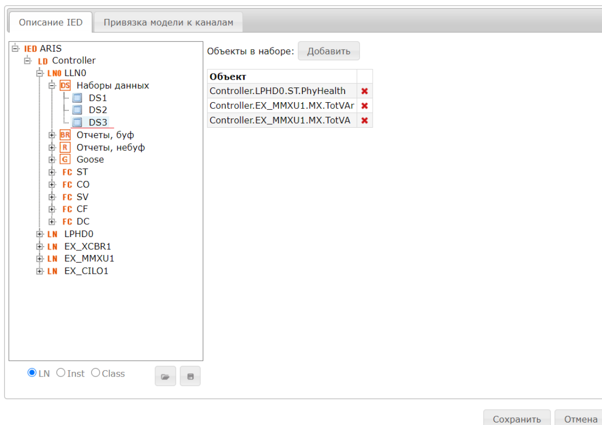
Рисунок 74 – Пример конфигурации набора данных в структуре IED
