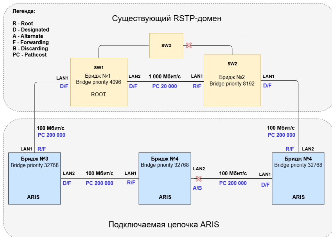
Рисунок 240 – Схема подключения цепочки из ARIS
