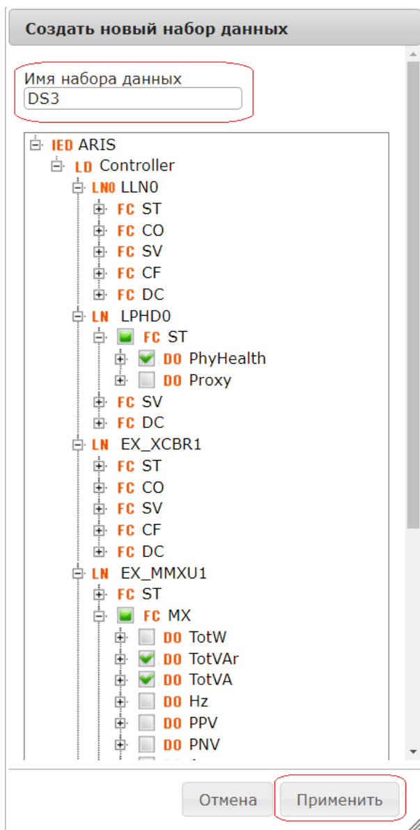
Рисунок 73 – Пример выборки данных в окне «Создать новый набор данных»
