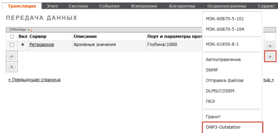
Рисунок 98 – Добавление сервера DNP3
