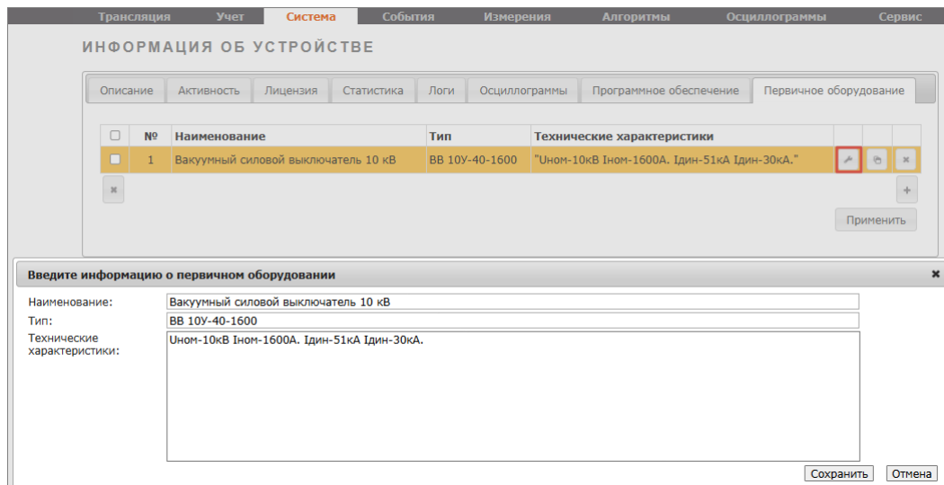
Рисунок 287 – Редактирование оборудования
