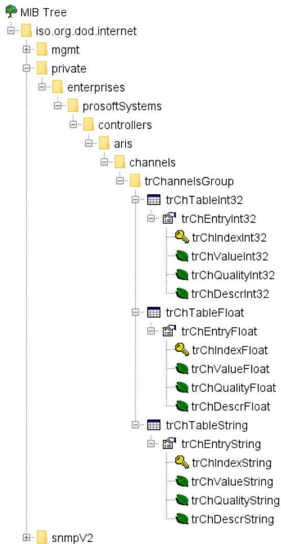
Рисунок 143 – Дерево «MIB»
