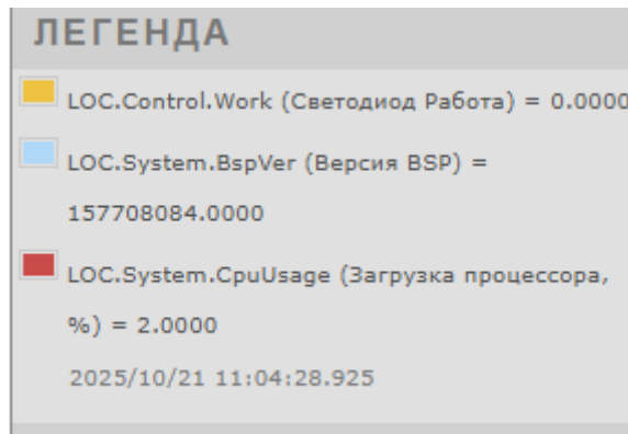
Рисунок 323 – Ретроархив «Легенда»
