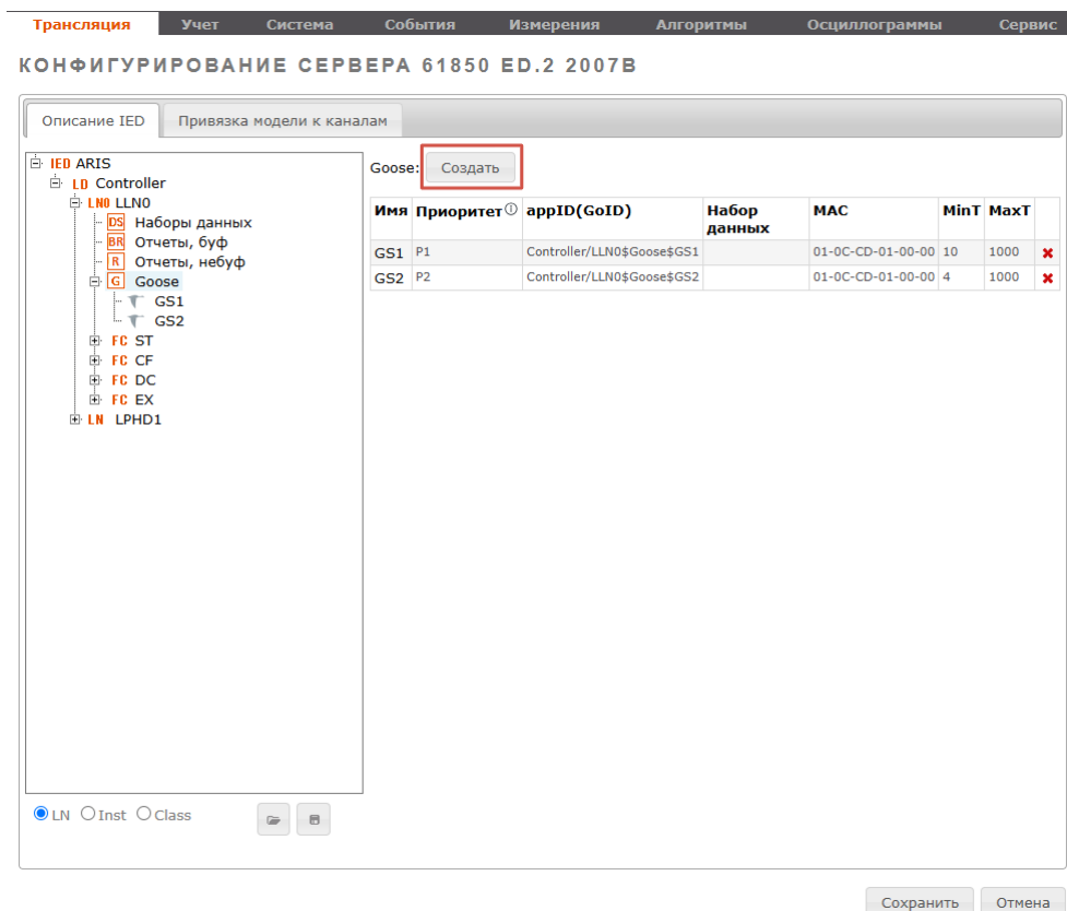
Рисунок 76 – Создание «GOOSE-сообщений»
