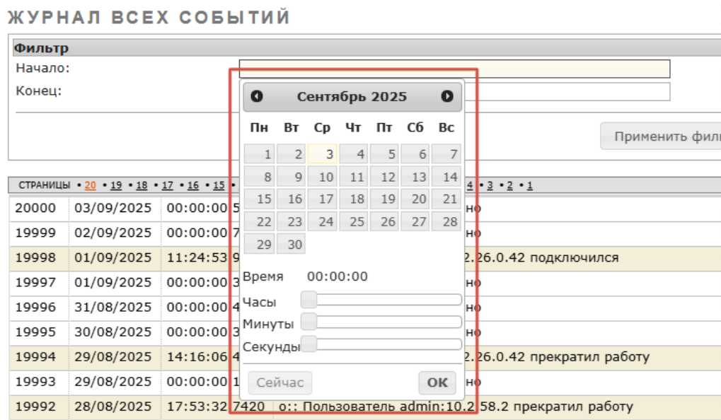
Рисунок 316 – Фильтр диапазона
