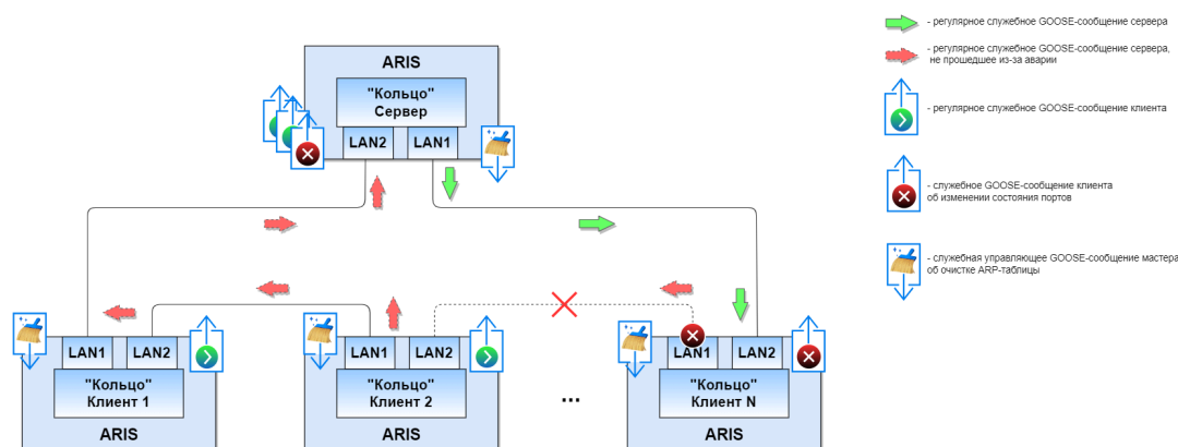
Рисунок 216 – Представление алгоритма работы в режиме «Кольцо»
