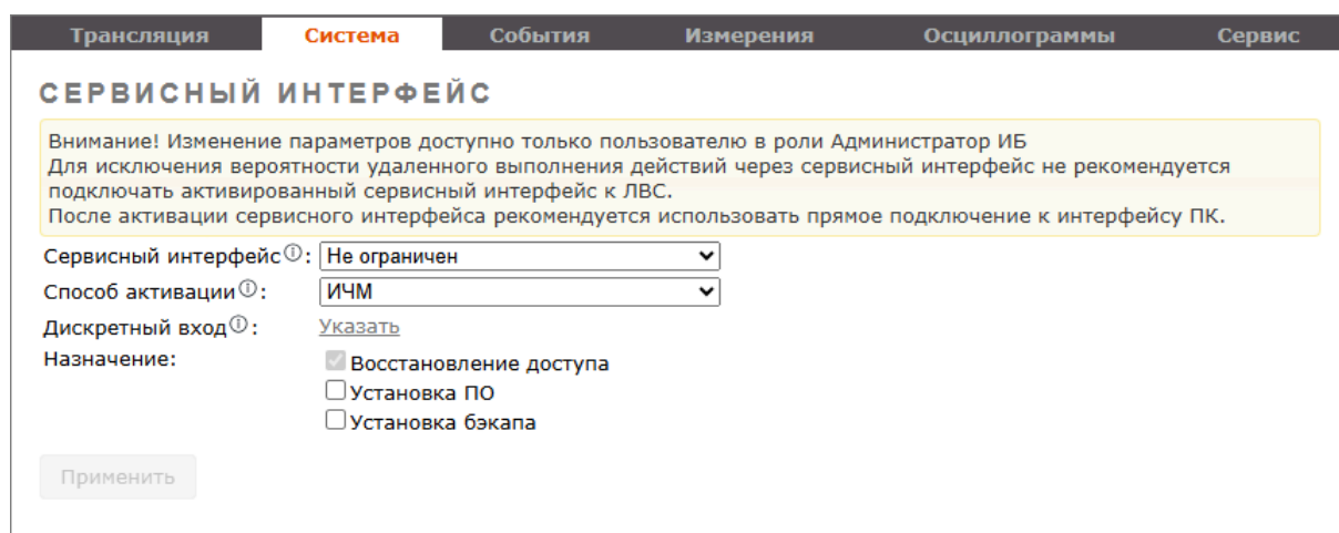
Рисунок 230 – Страница «Система» → «Сервисный интерфейс»
