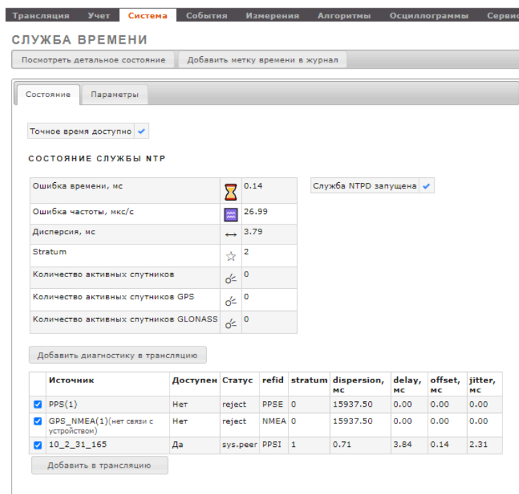
Рисунок 227 – Служба времени. Вкладка «Состояние»
