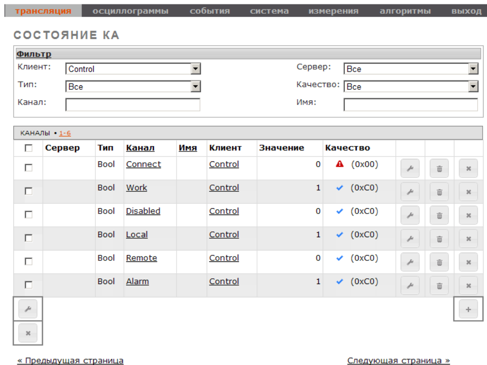
Рисунок 28 – Внутренние сигналы – Control
