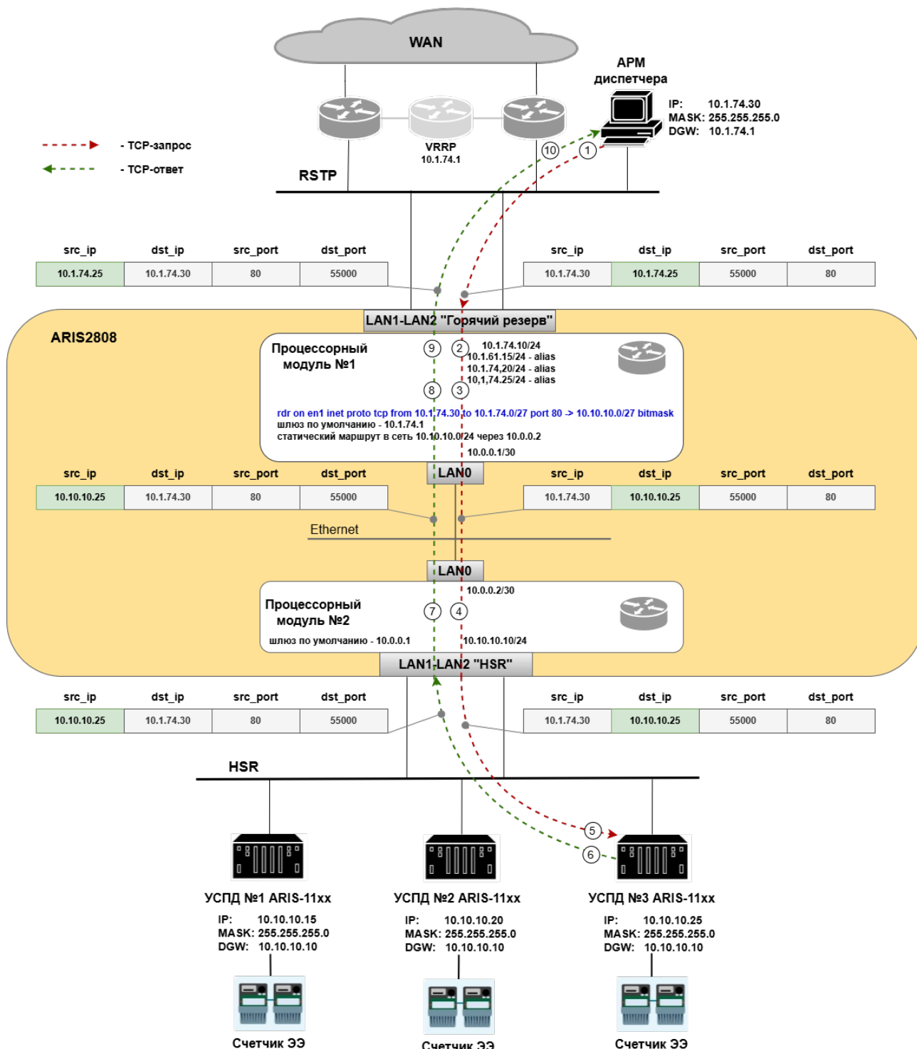
Рисунок 250 – Пример подключения АРМ диспетчера к УСПД со входящим NAT
