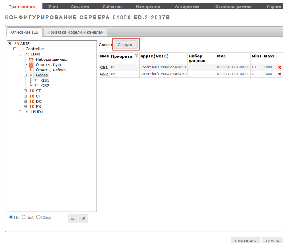
Рисунок 72 – Создание «GOOSE-сообщений»
