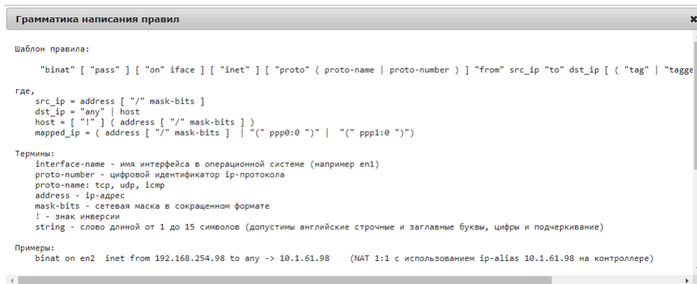
Рисунок 249 – Грамматика написания правил
