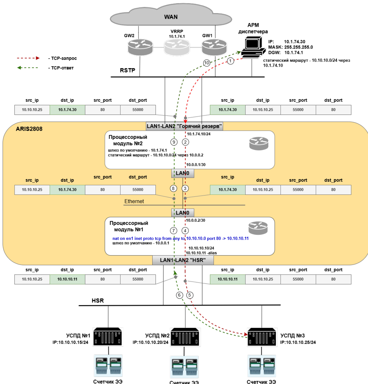
Рисунок 251 – Пример подключения АРМ диспетчера к УСПД с исходящим NAT
