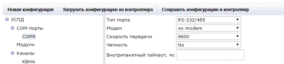
Рисунок 187 – Форма конфигурирования COM–порта
