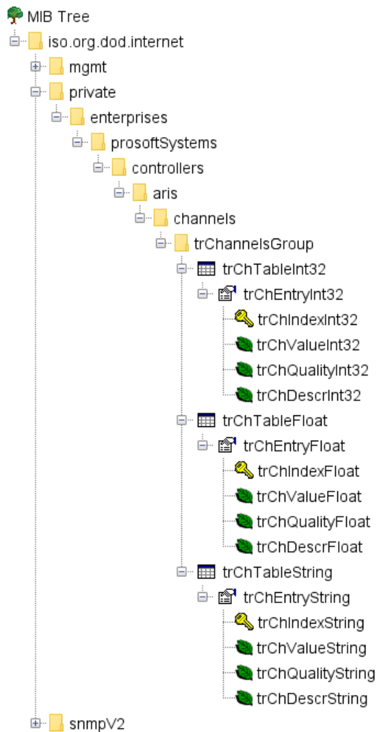
Рисунок 136 – Дерево «MIB»
