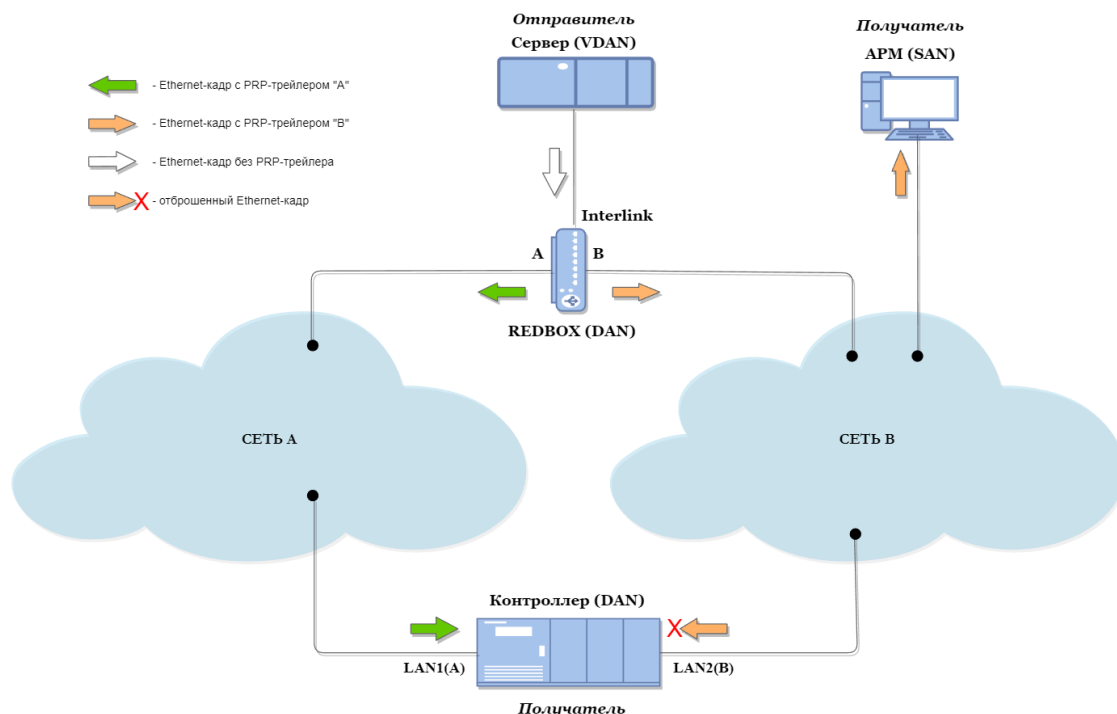
Рисунок 214 – Представление алгоритма работы в режиме резервирования «PRP»
