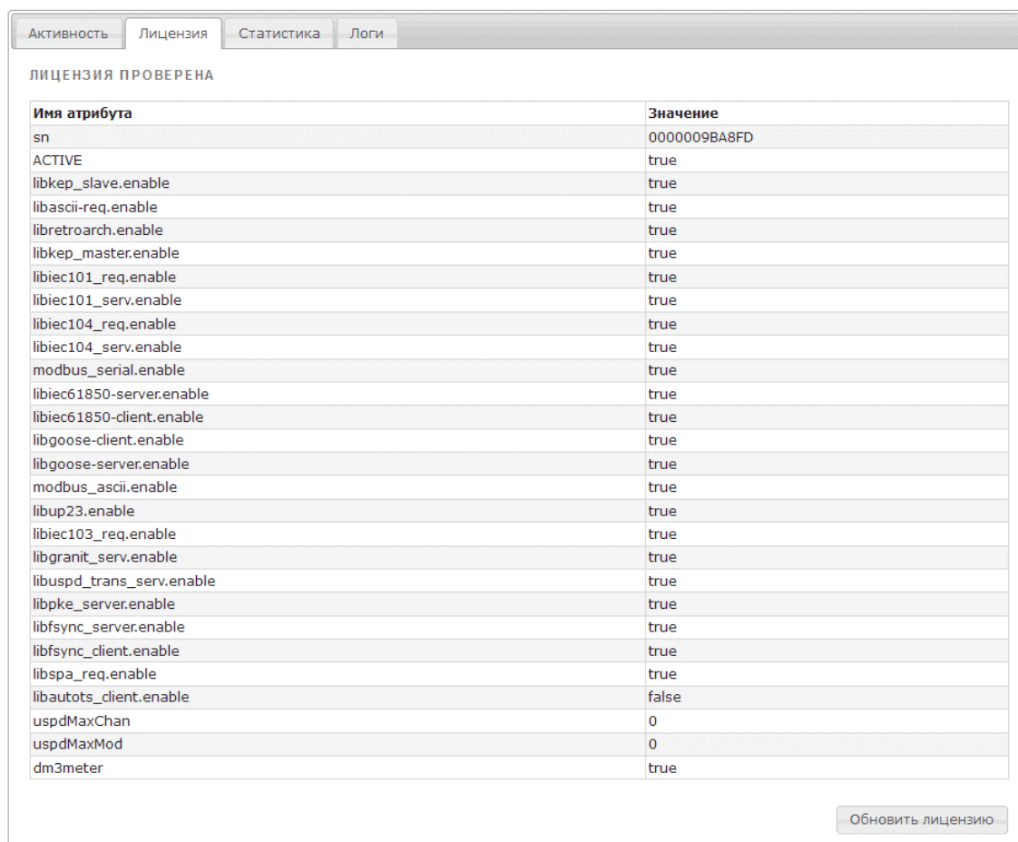
Рисунок 254 – Информация о системе (вкладка «Лицензия»)
