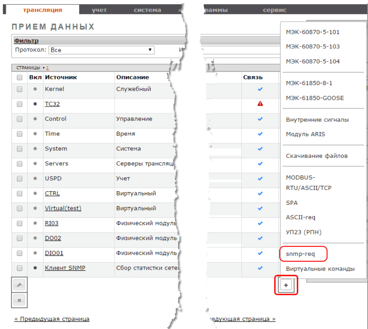
Рисунок 46 – Добавление клиента SNMP
