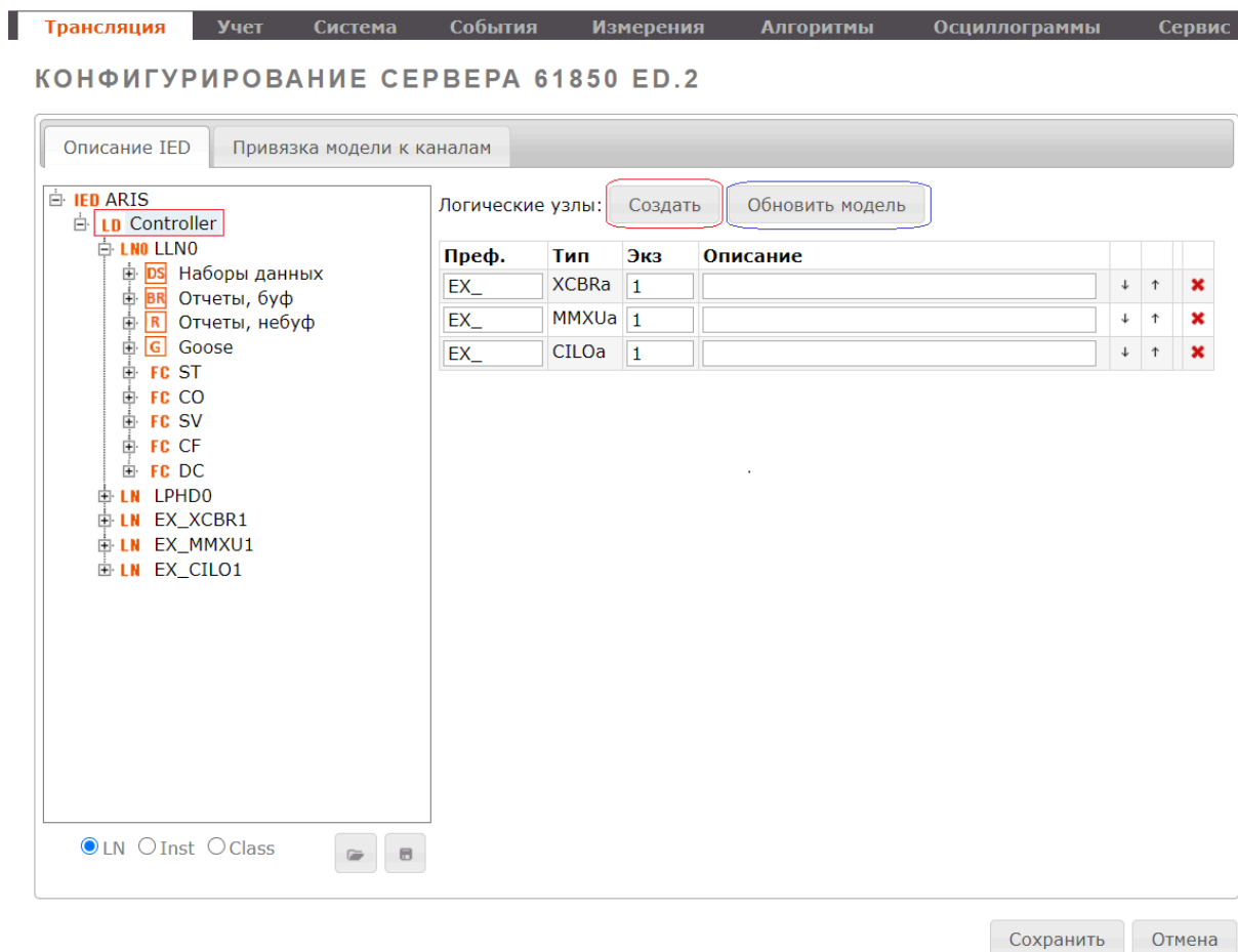
Рисунок 65 – Узел «Controller» в структуре IED
