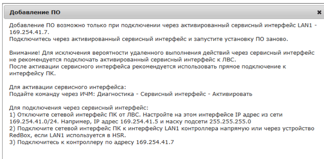
Рисунок 231 – Окно предупреждения активации сервисного интерфейса
