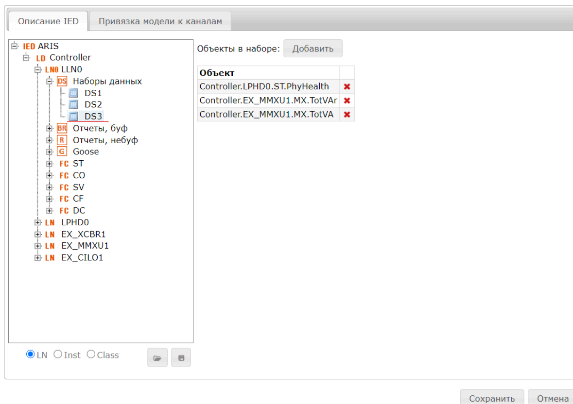
Рисунок 70 – Пример конфигурации набора данных в структуре IED
