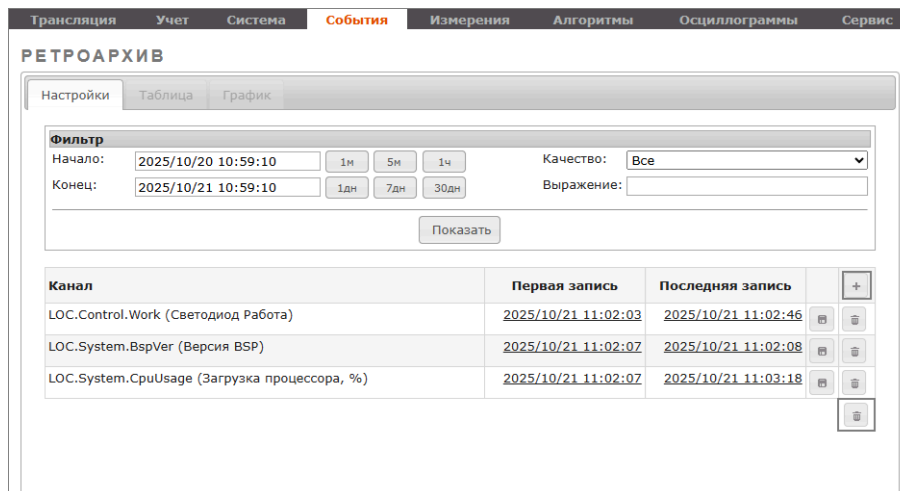
Рисунок 280 – Ретроархив. Вкладка «Настройки»
