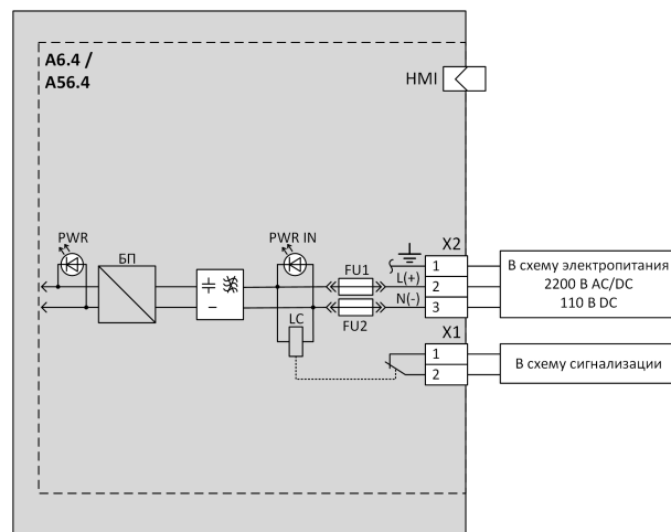
Рисунок 10 – Схема подключения модуля A5.4 Рисунок 11 – Схема подключения модуля A6.4
