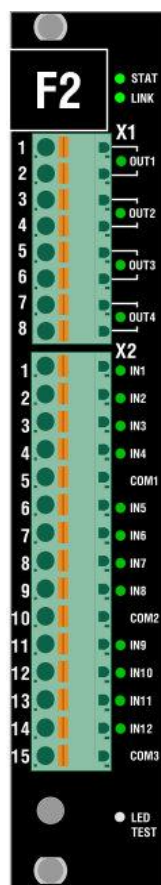
Рисунок 52 – Внешний вид модуля F2.4
