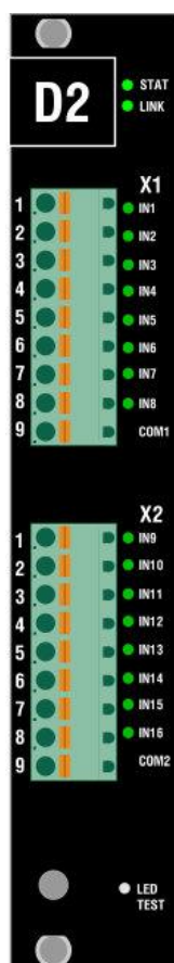
Рисунок 41 – Модуль D2.4 со стороны подключения внешних цепей
