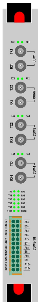
Рисунок 109 – Модуль Е5.6 со стороны подключения внешних цепей
