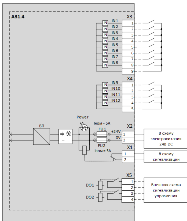
Рисунок 14 – Схема подключения модуля A31.4
