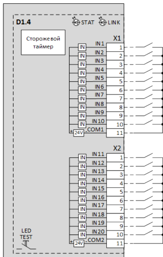
Рисунок 39 – Схема подключения дискретных входов с номинальным напряжением 24 В (1)
