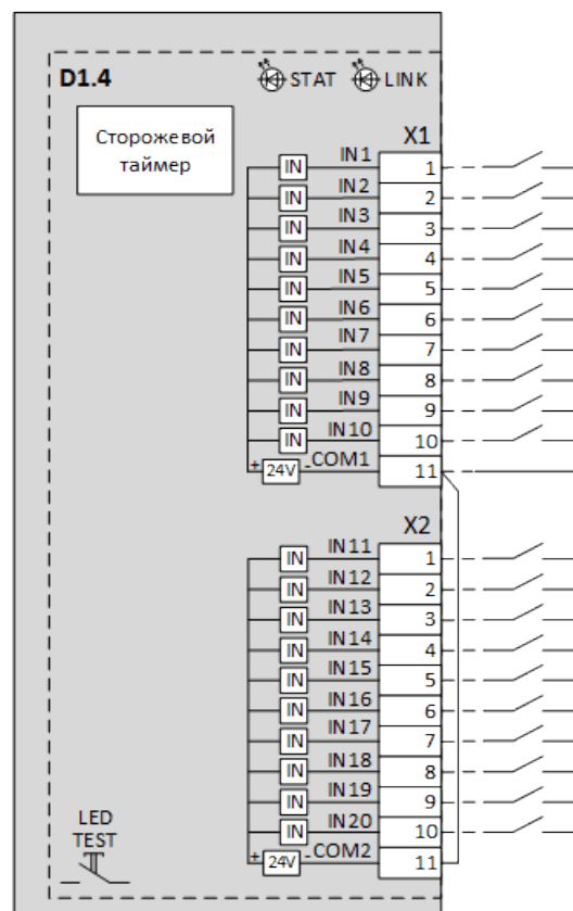
Рисунок 40 – Схема подключения дискретных входов с номинальным напряжением 24 В (2)
