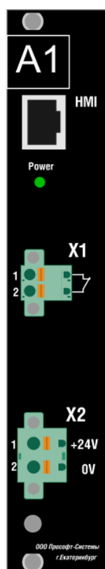
Рисунок 2 – Сторона подключения внешних цепей модуля A1.4
