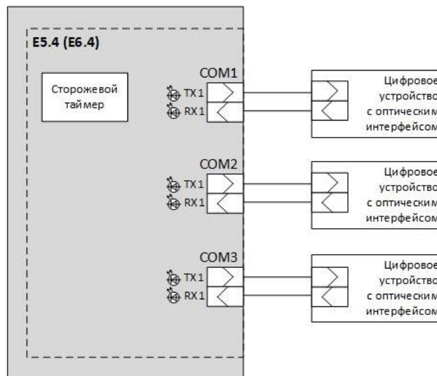
Рисунок 102 – Схема подключения внешних устройств к модулям E5.4, E6.4
