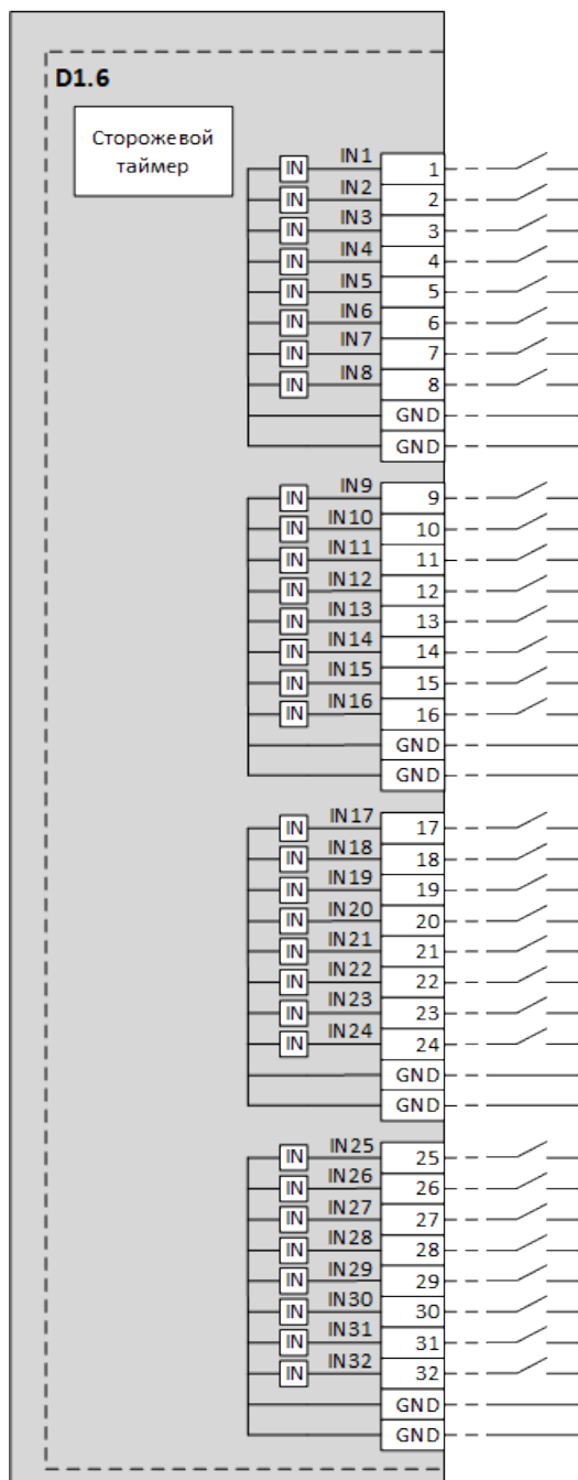
Рисунок 45 – Схема подключения дискретных входов с напряжением 24 В
