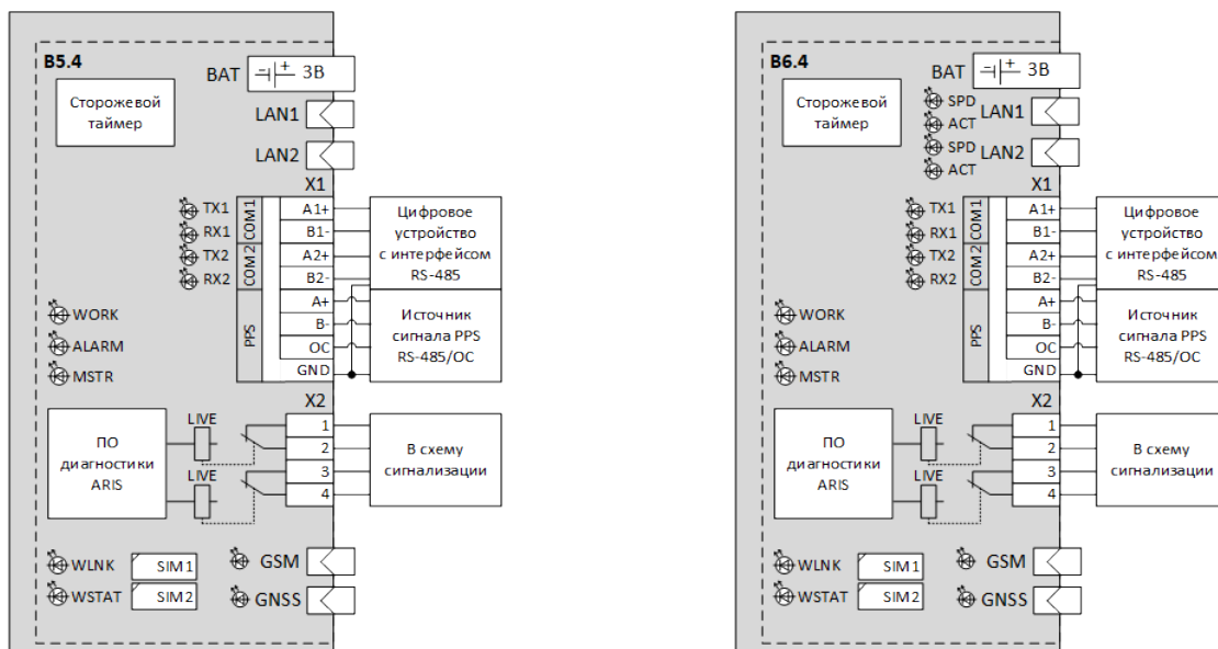
Рисунок 29 – Схема подключения модуля B5.4 Рисунок 30 – Схема подключения модуля B6.4
