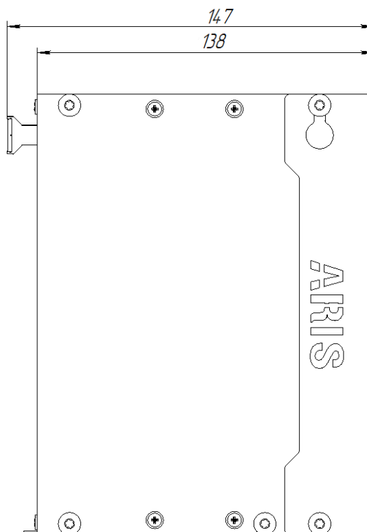
Рисунок Е.20 – Установочные размеры ARIS-4214, мм (вид сбоку)
