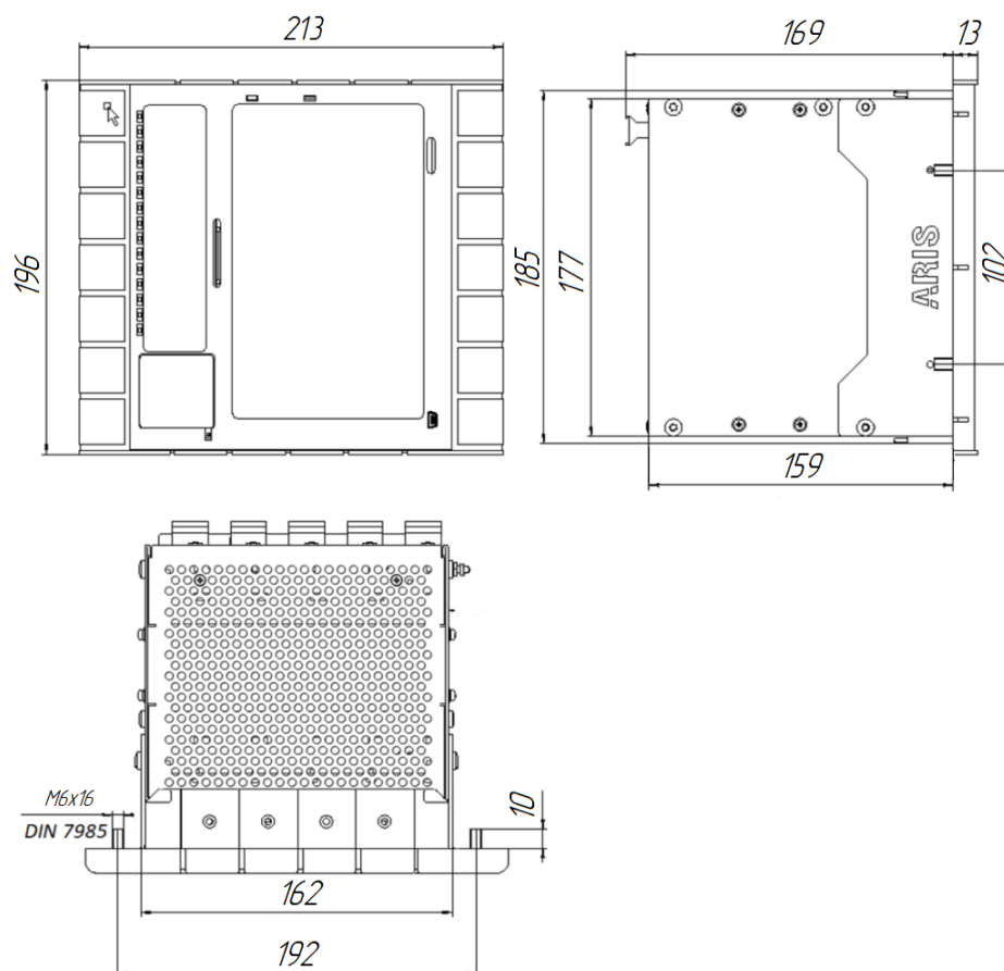
Рисунок Е.10 – Установочные размеры ARIS-4205 со встроенным ИЧМ, мм
