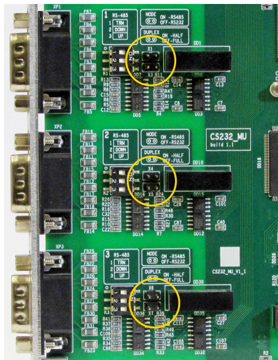
Рисунок 95 – Места размещения джамперов выбора режимов работы последовательных интерфейсов RS-232/422/485
