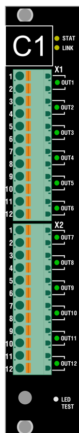
Рисунок 66 – Внешний вид модуля C1.4
