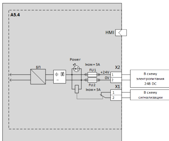
Рисунок 10 – Схема подключения модуля A5.4 Рисунок 11 – Схема подключения модуля A6.4
