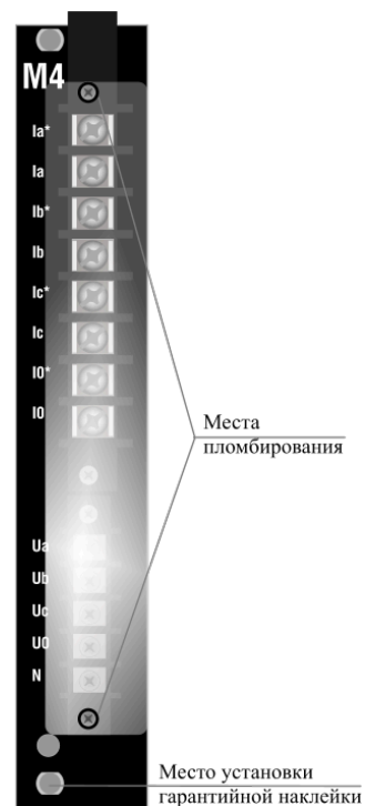
Рисунок 77 – Пломбировка разъемов модуля M4.4
