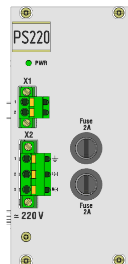
Рисунок 22 – Сторона подключения внешних цепей модуля A2.6
