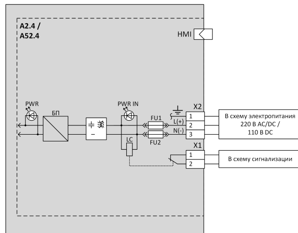
Рисунок 6 – Схема подключения модулей A2.4, A52.4
