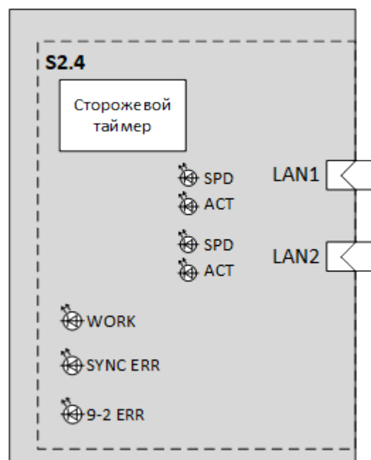
Рисунок 116 – Схема подключения модуля S2.4
