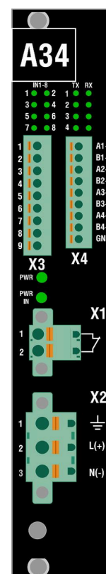
Рисунок 17 – Внешний вид модуля A34.4
