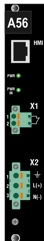
Рисунок 9 – Сторона подключения внешних цепей модуля А56.4
