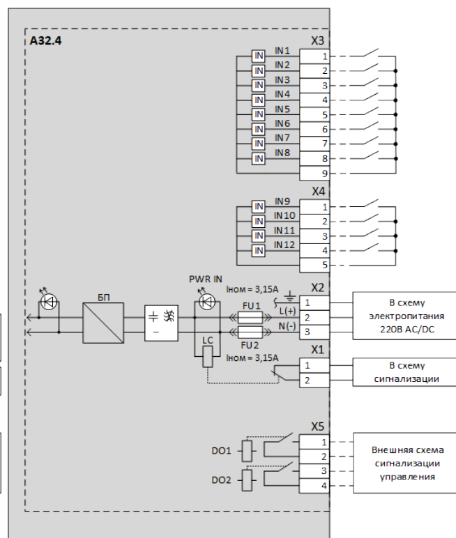
Рисунок 15 – Схема подключения модуля A32.4
