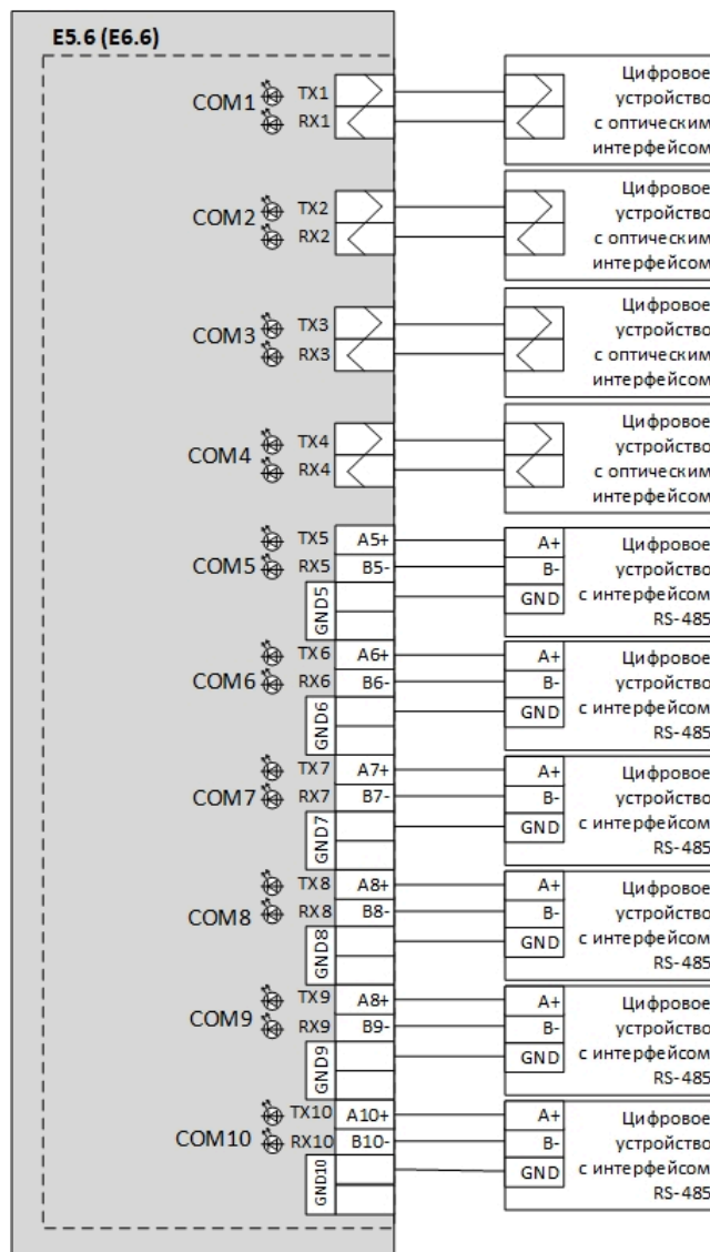
Рисунок 111 – Схема подключения внешних устройств к модулям E5.6, E6.6
