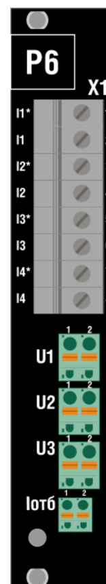
Рисунок 118 – Сторона подключения внешних цепей модуля Р6.4 (сторона подключения внешних цепей модуля Р7.4 имеет аналогичный вид лицевой панели)
