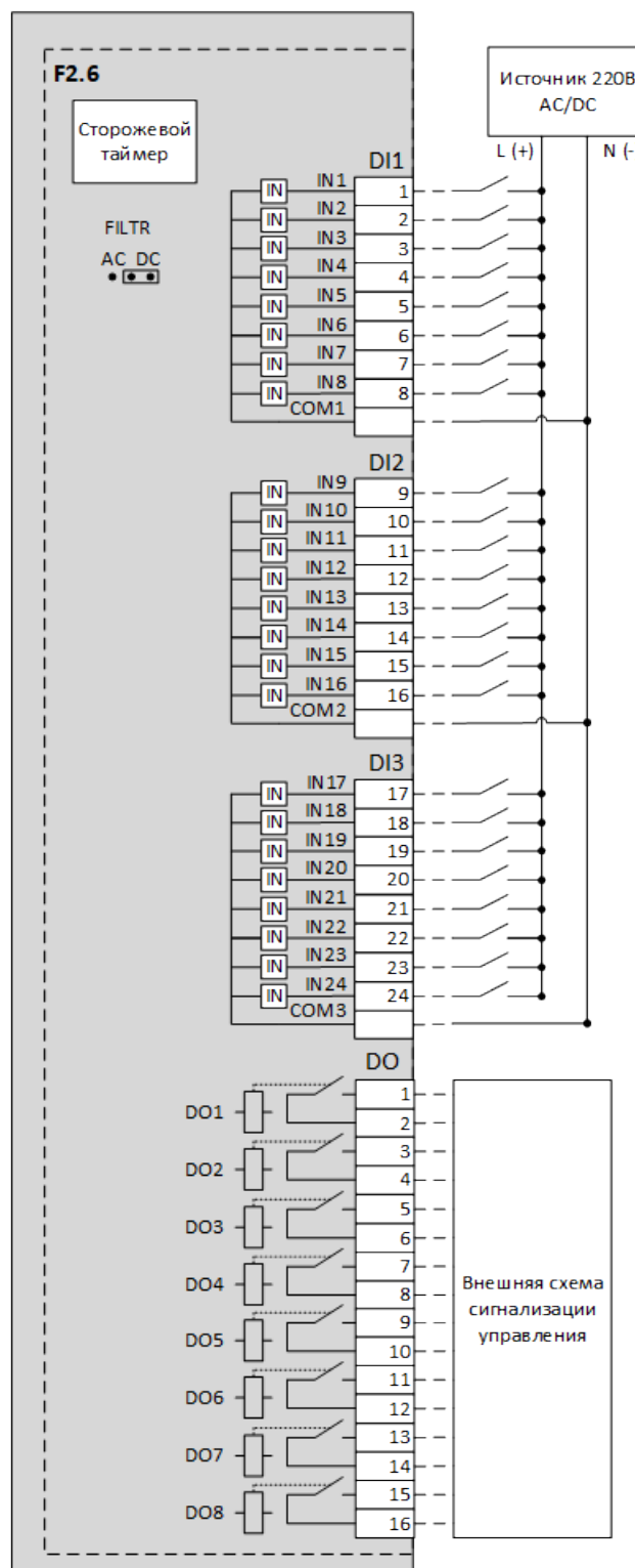
Рисунок 63 – Схема подключения дискретных входов/выходов модуля F2.6 с напряжением на разомкнутых клеммах 220 В
