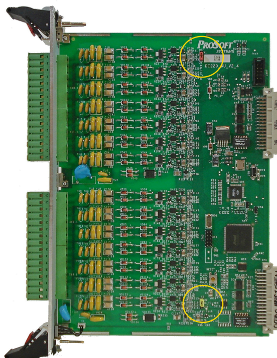
Рисунок 48 – Размещение джамперов Filtr модуля
