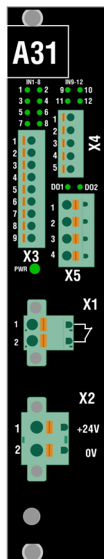
Рисунок 12 – Внешний вид модуля A31.4
