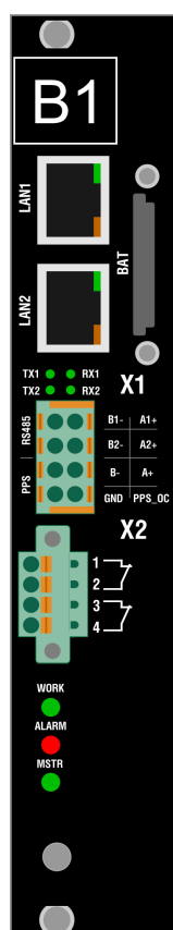
Рисунок 23 – Внешний вид модуля B1.4
