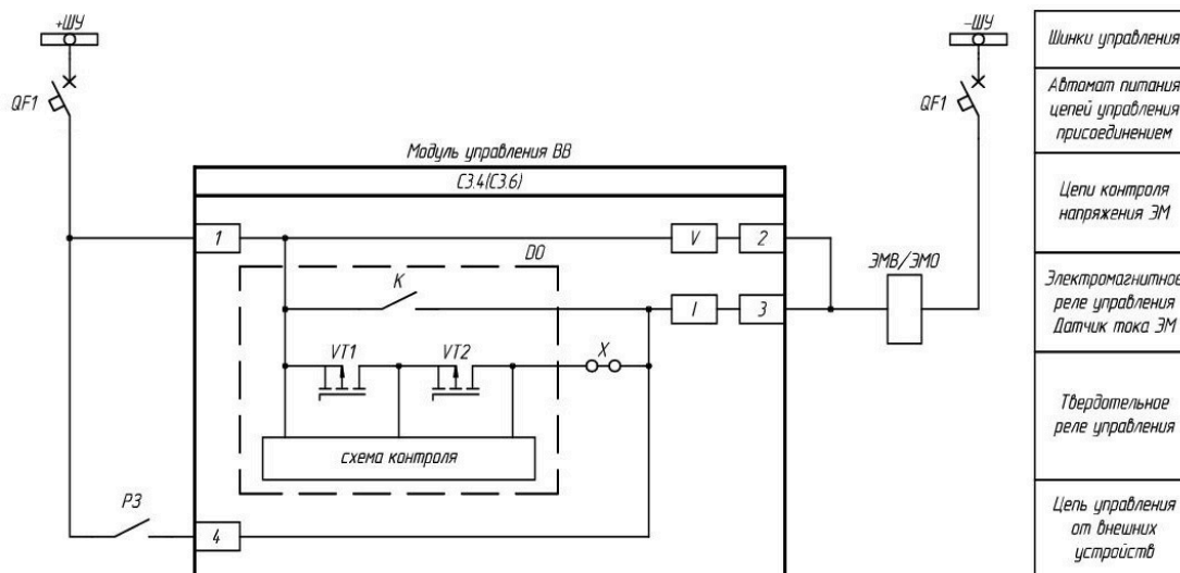
Рисунок 71 – Схема подключения модуля
