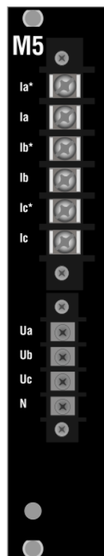
Рисунок 80 – Сторона подключения внешних цепей модуля M5.4
