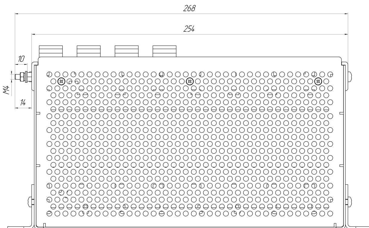
Рисунок Е.14 – Установочные размеры ARIS-4208, мм (вид сверху)
