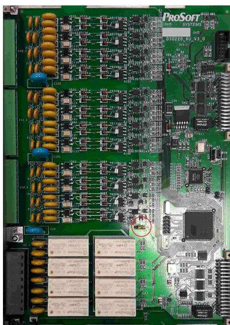
Рисунок 64 – Размещение джампера "Filtr" модуля F2.6
