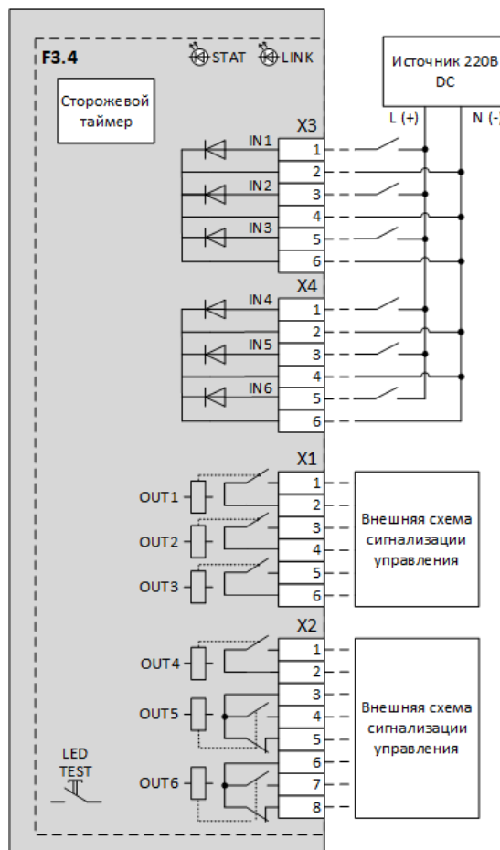
Рисунок 56 – Схема подключения внешних цепей модуля дискретных входов/выходов F3.4
