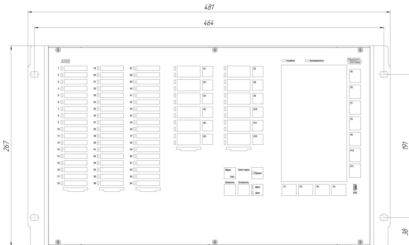
Рисунок Е.26 – Установочные размеры ARIS-4212, мм (вид спереди)
