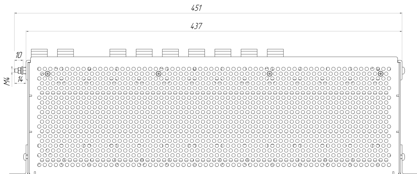
Рисунок Е.21 – Установочные размеры ARIS-4214, мм (вид сверху)
