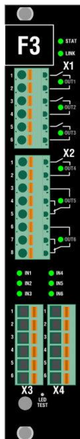
Рисунок 55 – Внешний вид модуля F3.4
