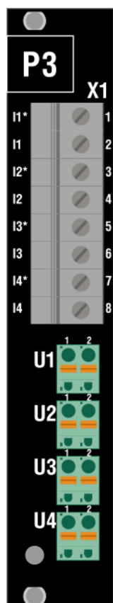
Рисунок 117 – Сторона подключения внешних цепей модуля Р3.4 (сторона подключения внешних цепей модуля Р4.4 имеет аналогичный вид)
