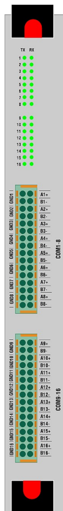
Рисунок 104 – Вид передней панели модуля E1.6
