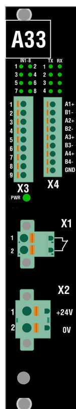
Рисунок 16 – Внешний вид модуля A33.4
