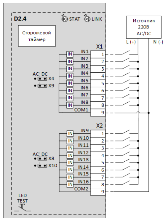
Рисунок 42 – Схема подключения дискретных входов с номинальным напряжением 220 В (переменного/постоянного тока)
