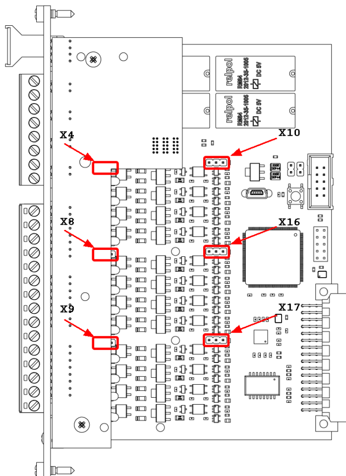
Рисунок 54 – Расположение перемычек модуля
