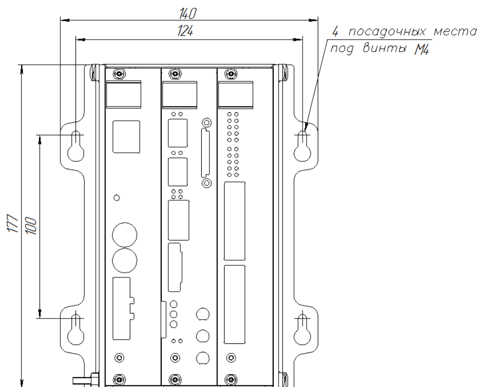
Рисунок Е.3 – Установочные размеры ARIS-4203, мм (вид сверху)
