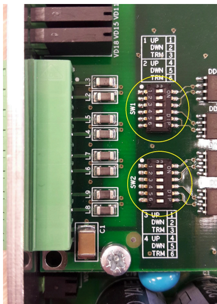
Рисунок 20 – Размещение групповых движковых переключателей SW1, SW2
