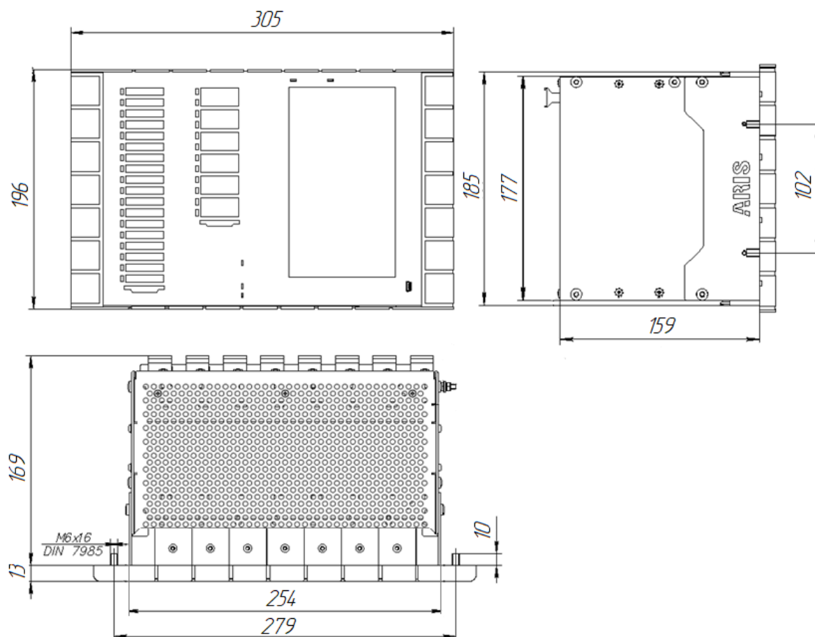
Рисунок Е.17 – Установочные размеры ARIS-4208 со встроенным ИЧМ, мм
