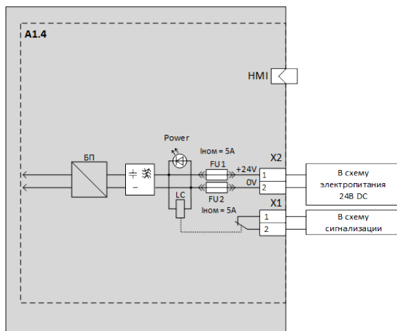
Рисунок 5 – Схема подключения модуля A1.4
