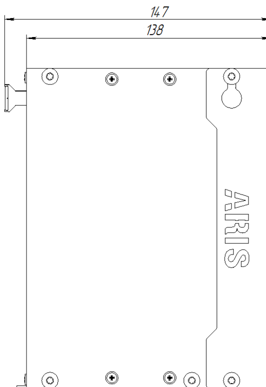
Рисунок Е.2 – Установочные размеры ARIS-4203, мм (вид сбоку)
