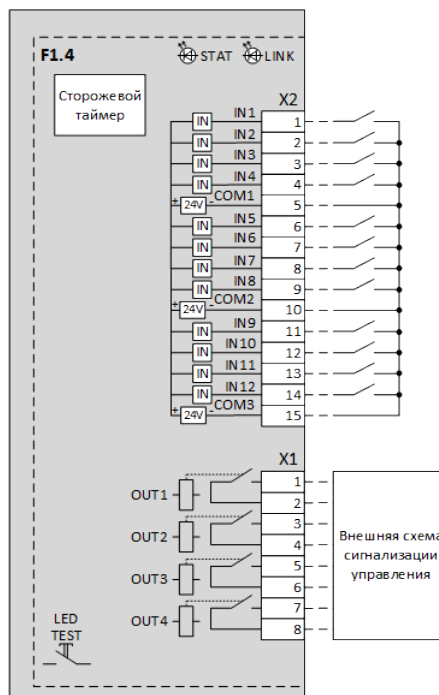
Рисунок 51 – Схема подключения модуля дискретных входов/выходов F1.4
