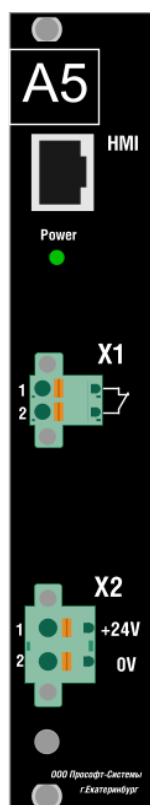
Рисунок 7 – Сторона подключения внешних цепей модуля А5.4
