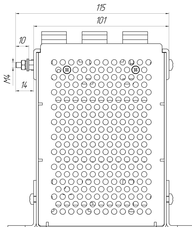
Рисунок Е.3 – Установочные размеры ARIS-4203, мм (вид сверху)
