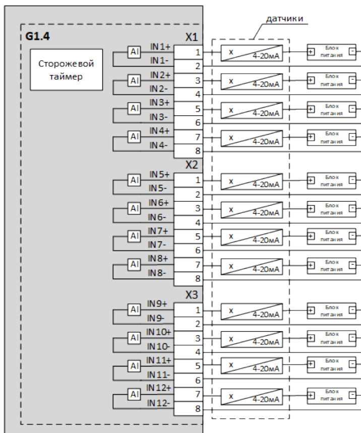
Рисунок 86 – Схема подключения внешних устройств к модулю G1.4
