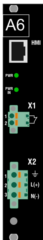
Рисунок 8 – Сторона подключения внешних цепей модуля А6.4
