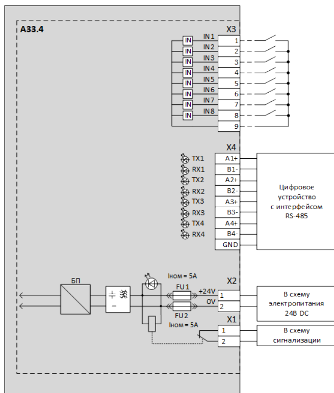
Рисунок 18 – Схема подключения модуля A33.4
