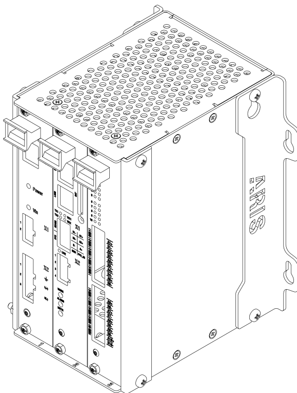
Рисунок Е.1 – Общий вид ARIS-4203
