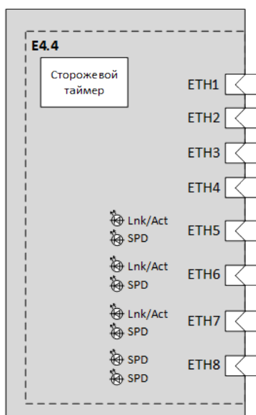
Рисунок 99 – Схема подключения внешних устройств к модулю E4.4
