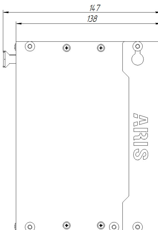
Рисунок Е.6 – Установочные размеры ARIS-4205, мм (вид сбоку)
