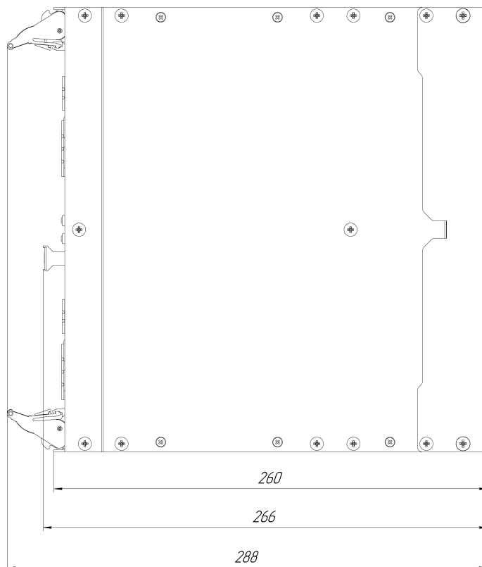
Рисунок Е.27 – Установочные размеры ARIS-4212, мм (вид сбоку)
