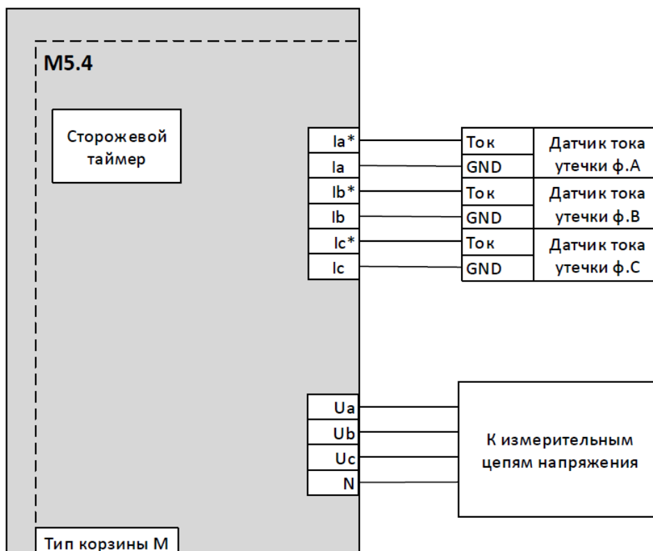
Рисунок 82 – Схема подключения внешних цепей к модулю M5.4
