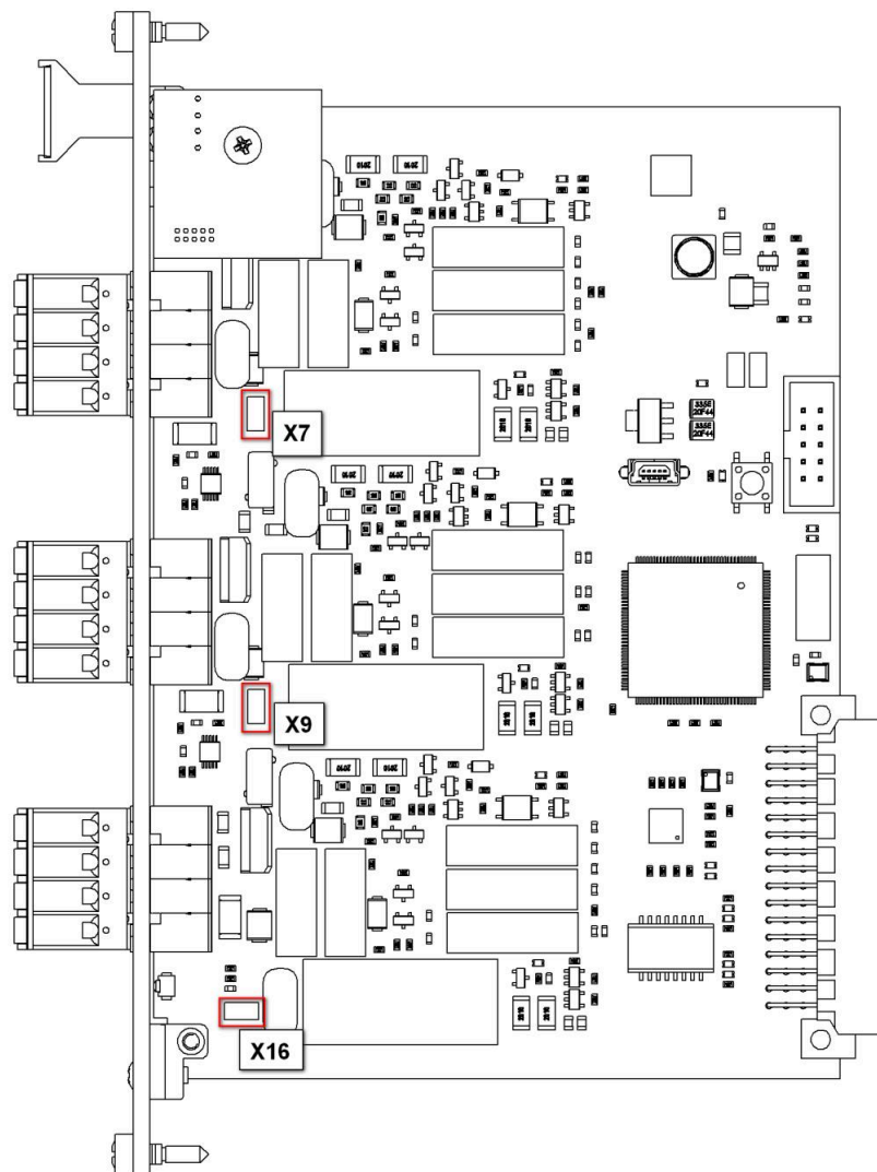
Рисунок 73 – Места размещения джамперов подключения или вывода из работы твердотельных реле по отдельным каналам
