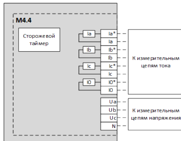
Рисунок 79 – Схема подключения модуля M4.4
