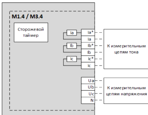
Рисунок 78 – Схема подключения модулей M1.4, M3.4
