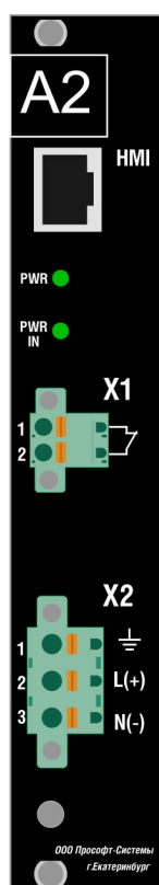
Рисунок 3 – Сторона подключения внешних цепей модуля A2.4
