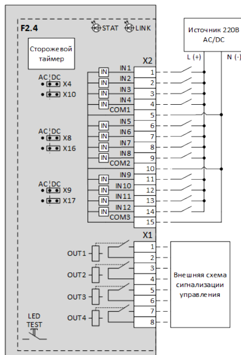
Рисунок 53 – Схема подключения дискретных входов/выходов модуля F2.4
