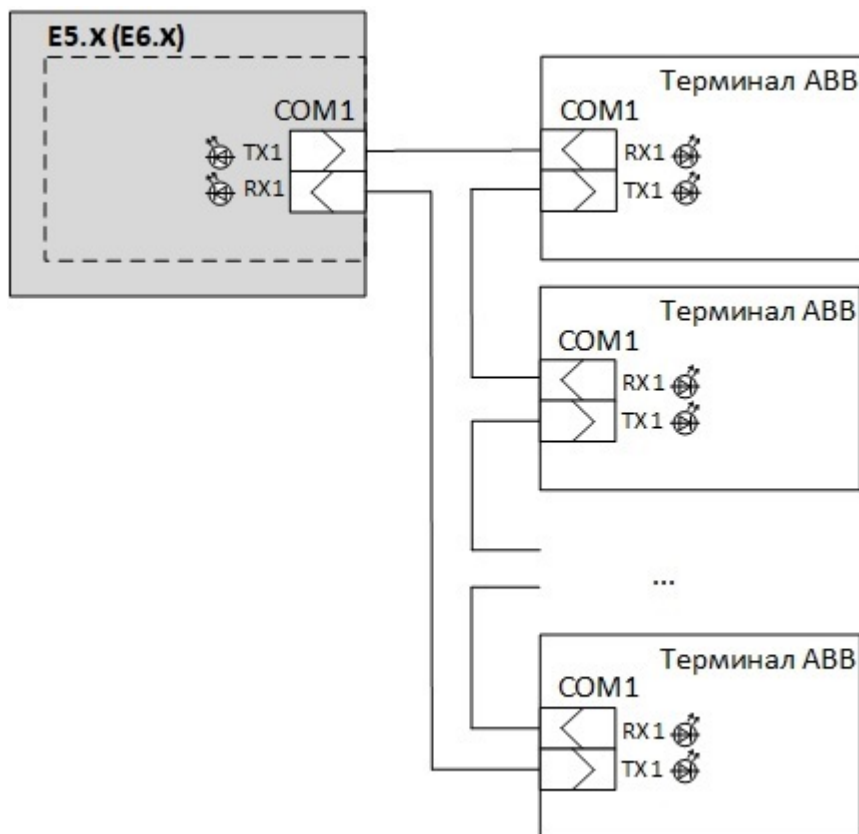
Рисунок 103 – Пример схемы подключения внешних устройств
