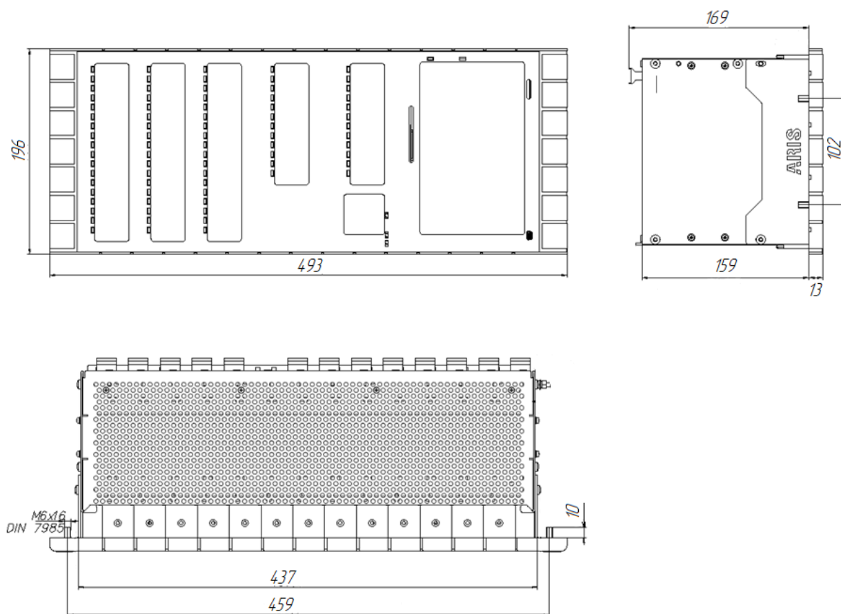
Рисунок Е.24 – Установочные размеры ARIS-4214 со встроенным ИЧМ, мм
