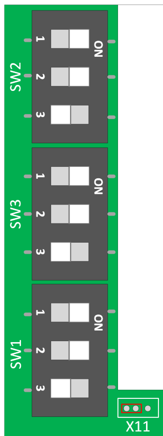
Рисунок 36 – Состояние по умолчанию группового движкового переключателя
