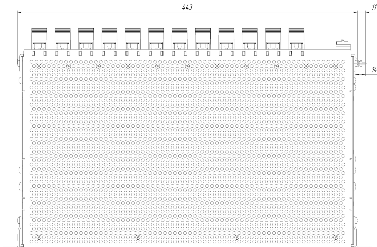
Рисунок Е.28 – Установочные размеры ARIS-4212, мм (вид сверху)
