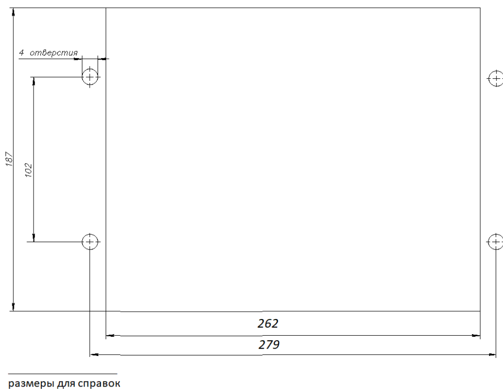
Рисунок Е.18 – Установочные размеры монтажного окна ARIS-4208 при врезке в панель, мм
