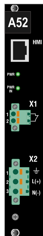
Рисунок 4 – Сторона подключения внешних цепей модуля A52.4
