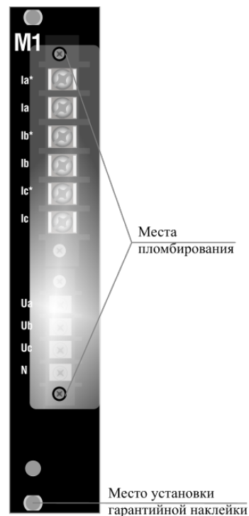
Рисунок 75 – Пломбировка разъемов модуля M1.4 (M3.4)
