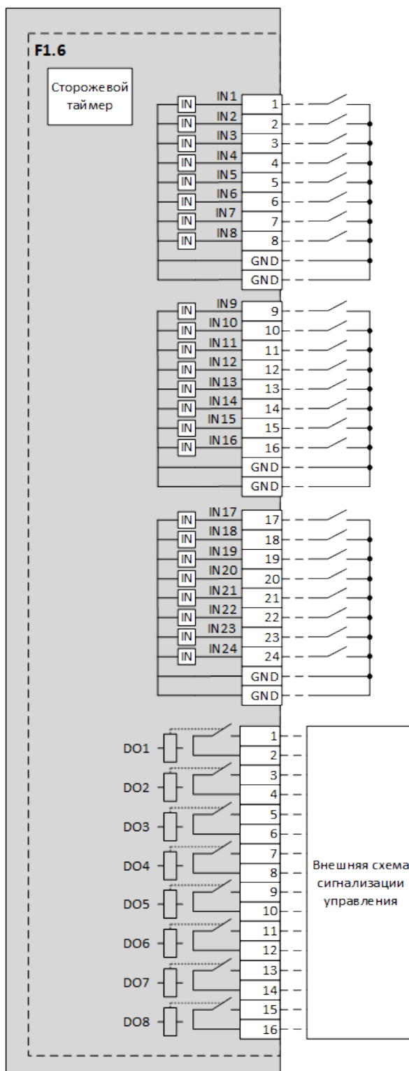
Рисунок 61 – Схема подключения модуля F1.6 дискретных входов/выходов с номинальным напряжением на разомкнутом контакте 24 В
