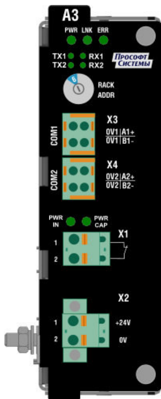
Рисунок 11 – Внешний вид модуля АЗ.1
