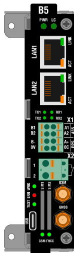
Рисунок 16 – Сторона подключения внешних цепей модуля B5.1
