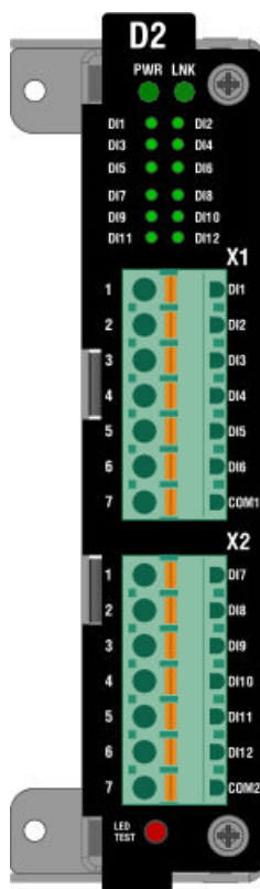
Рисунок 25 – Сторона подключения внешних цепей модуля D2.1
