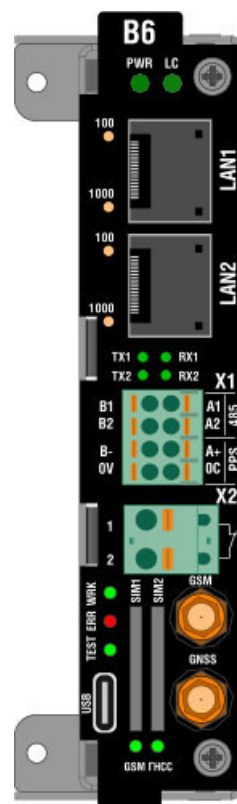
Рисунок 18 – Сторона подключения внешних цепей модуля B6.1
