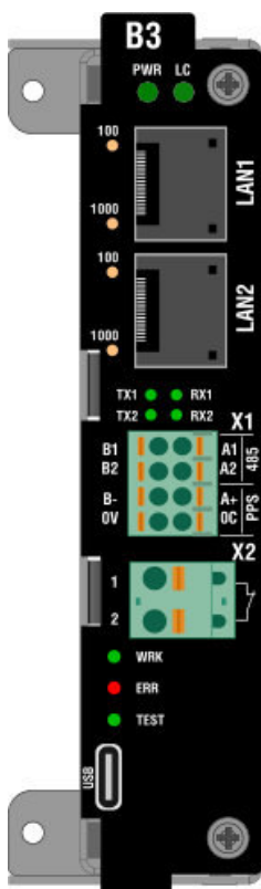
Рисунок 17 – Сторона подключения внешних цепей модуля B3.1
