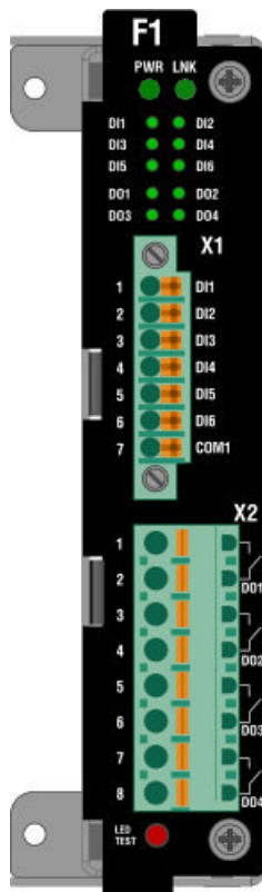
Рисунок 27 – Сторона подключения внешних цепей модуля F1.1
