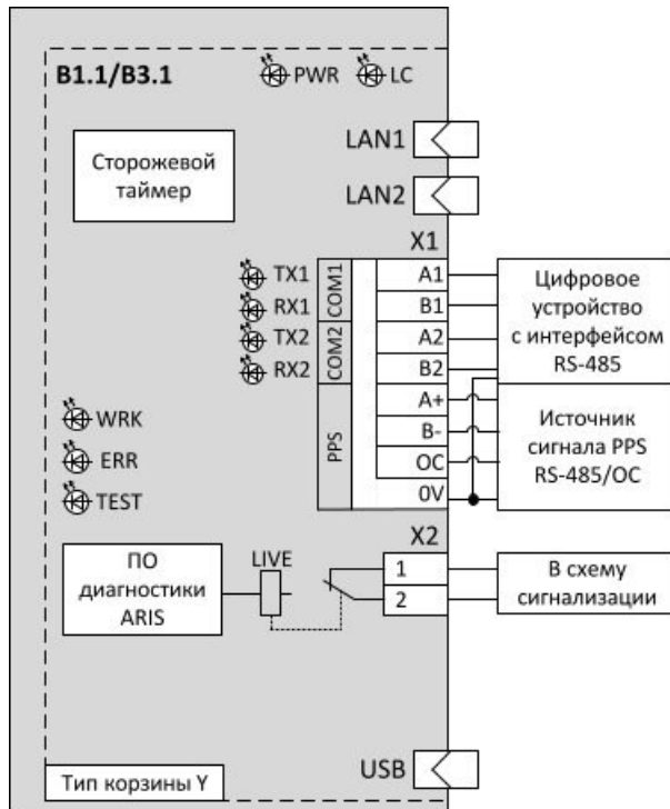
Рисунок 19 – Схема подключения модуля процессорного B1.1, B3.1
