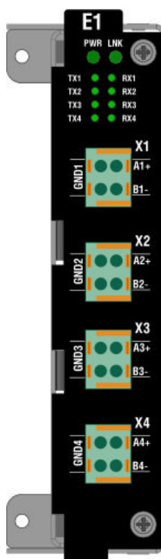
Рисунок 35 – Внешний вид модуля Е1.1
