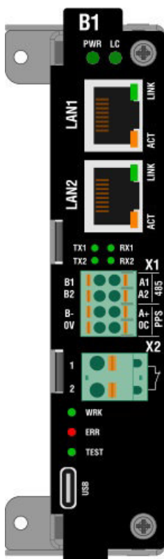
Рисунок 15 – Сторона подключения внешних цепей модуля B1.1
