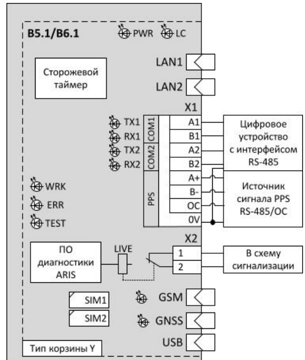
Рисунок 20 – Схема подключения модуля процессорного B5.1, B6.1
