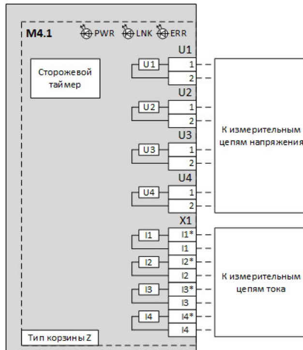
Рисунок 34 – Схема подключения модуля М4.1
