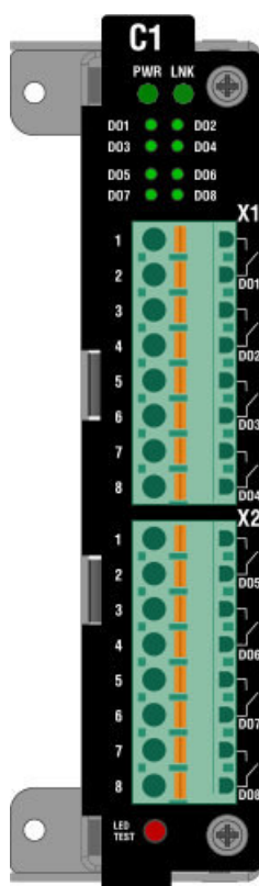
Рисунок 31 – Сторона подключения внешних цепей модуля C1.1
