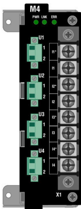
Рисунок 33 – Внешний вид модуля М4.1
