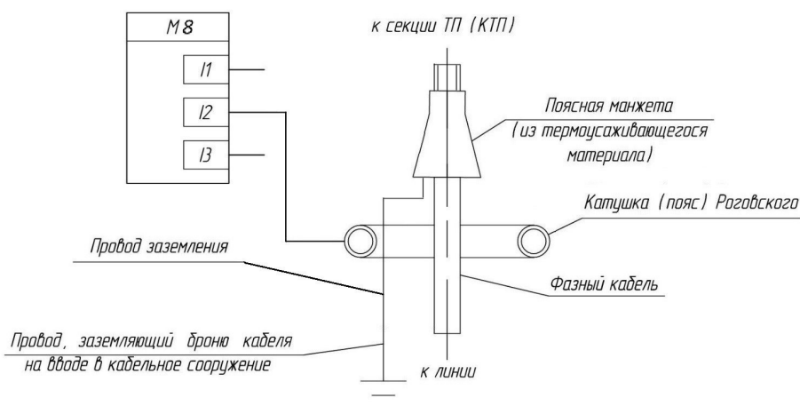
Рисунок М.3 – Установка КР на кабель до концевой муфты
